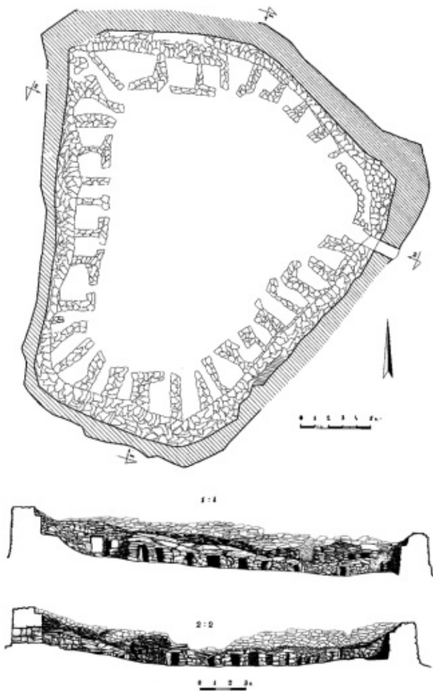
სურ. 75. ჯავახეთი. შაორის კომპლექსის ცენტრალური ნაწილის გეგმა (შეადგინეს ა. თევზაძემ, შ. მელიქიძემ, გ. ნარიმანიშვილმა).
