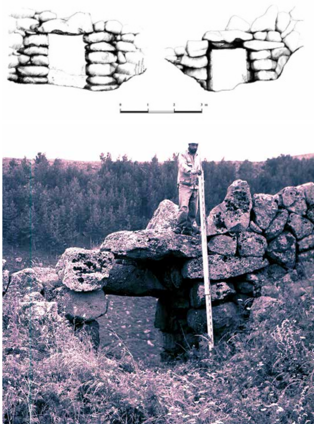
სურ. 131. თრიალეთი. თეზი /ავრანლო. ზედა სიმაგრე. კარიბჭე (ჩანახატი შ. მელიქიძის).
