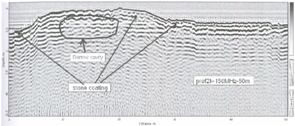
ნახ. 2. იგივე რადაროგრამა რელიეფის შესწორების გათვალისწინებით. განიერი ისრით ნაჩვენებია შესაძლო სიღრუვის მდებარეობა (შემოკონტურულია), ისრებით გამოკვეთილია ლოდებით მდებარეობა (შემოფენა).
