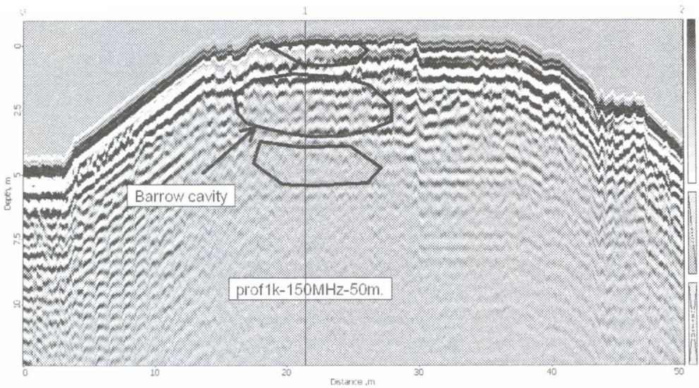
ნახ. 4. იგივე რადაროგრამა, რაც ნახ. 3 არის ნაჩვენები, რელიეფზე შესწორების შეტანის შემდეგ. ისრით მითითებულია და წრეებით შემოფარგლულია ყორღანში არსებული (საეარაუდო) სიღრუეები.
