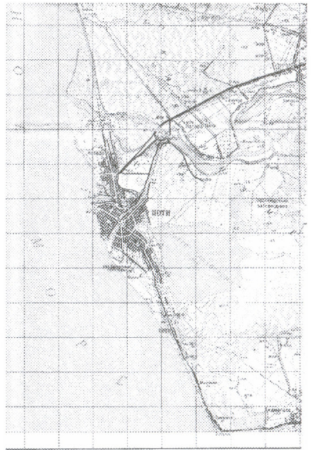
სურ. 3. თანამედროვე ფოთის და პალიასტომის ტბის ტოპოგრაფიული გეგმა.
