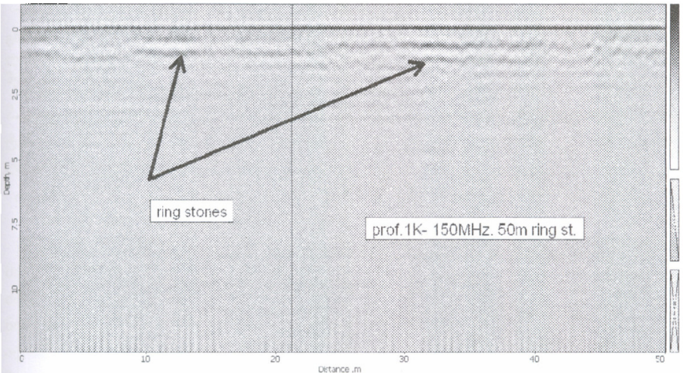
ნახ. 3. წარმოდგენილია ნახაზებზე 1, 2-ზე მოტანილი რადაროგრამის მართობულ პროფილზე მიღებული რადაროგრამა. ისრებით ნაჩვენებია წრეულად განლაგებული ყორღანული ლოდნარი.
