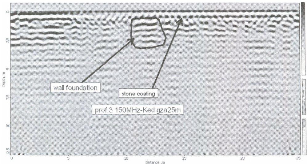
ნახ. 5. წარმოდგენილია შირაქის ნაქალაქარის 450-მეტრიანი მონაკვეთის გეორადარული ჭრილი. გამოიყო გეორადარული ფენები. ისინი მდებარეობენ: პირველი 1-1.5 მ, მეორე 2-2.5 მ. ჭრილის გასწვრივ გამოიყო გრუნტის წყლის დონე 1-1.5 მ. (მუქი შავი ზოლი) და განყლოვანების უბანი რადაროგრამის ბოლოს 420-450 მ. ზედაპირთან ახლო ისრებით მინიშნებულ ადგილებზე (საეარაუდოდ) ფუნდამენტის ნარჩენებია.
