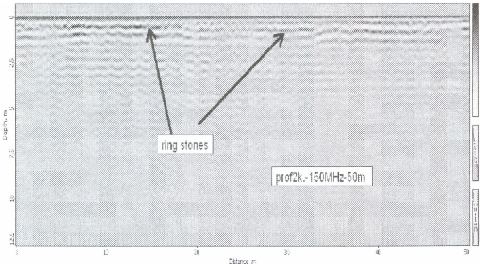
ნახ. 1. რადაროგრამაზე ყორღანის (სავარაუდოდ) წრიულად (ჭრილში) განლაგებული ლოდებია. რადარული სიგნალის ჩაღწევის სიღრმე - 10 მ. ნახატებზე 1-6 მოცემულია: ყ-ღერძზე სიღრმე მეტრებში, ხ-ღერძზე – მანძილი პროფილის გასწვრივ მეტრებში.
