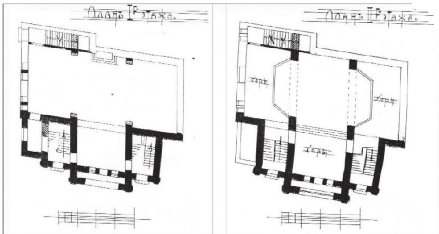
სურ. 1. აშქენაზების სინაგოგა. განუხორციელებელი პროექტი. სართულის გეგმები. 1913
