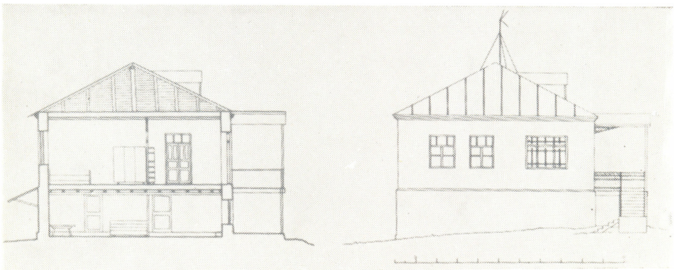
სურ. 2. ახალციხის რ-ნი. სოფ. ივლიტა. თამაზაშვილის სახლის კრილი და ფასადი.
