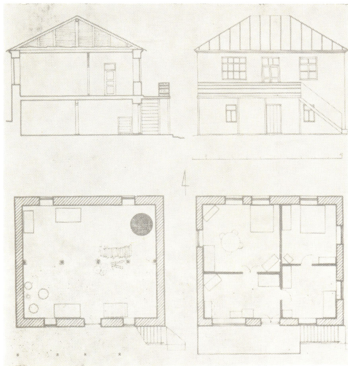
სურ. 1. ახალციხის რ-ნი სოფ. მუსხი. ლადუი საეის ძე ქურდაძის სახლის გეგმები, ჭრილი და ფასადი
