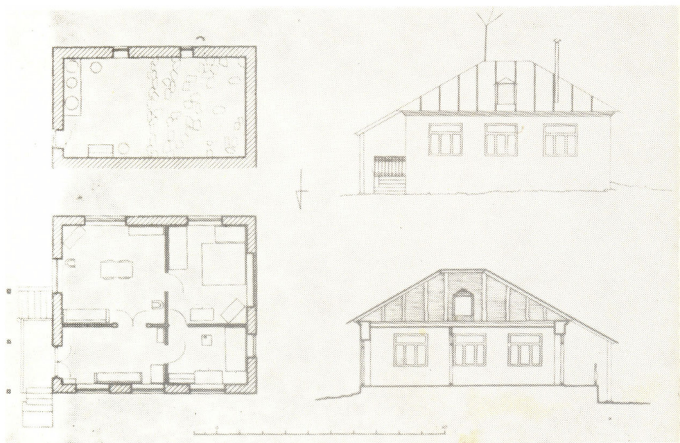
სურ. 2. სოფ. კლდე. ტოგო გრიგოლის ძე კაპანაძის სახლის გეგმა, ფასადი და ჭრილი.
