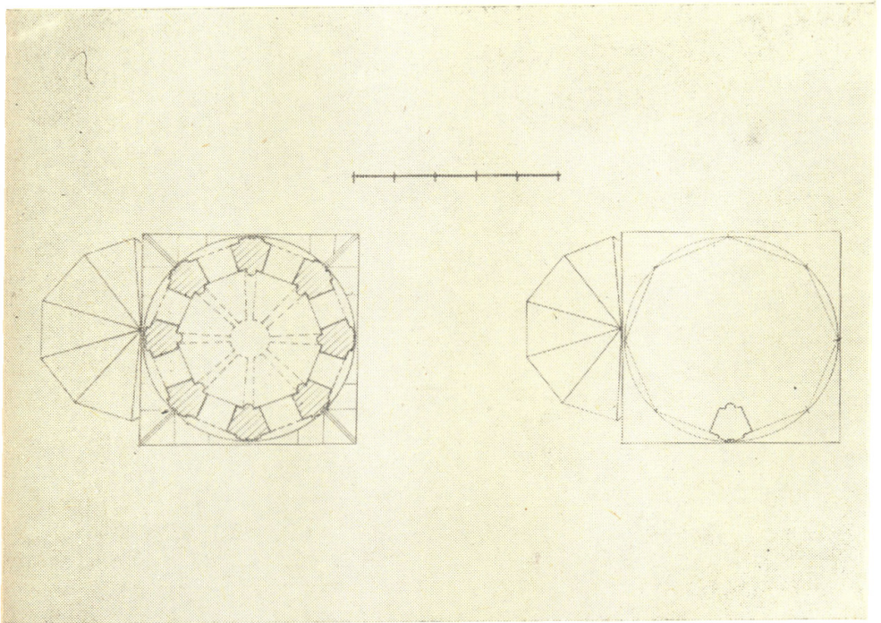
სურ. 7. მეორე იარუსის გეგმის რესტავრაცია.
