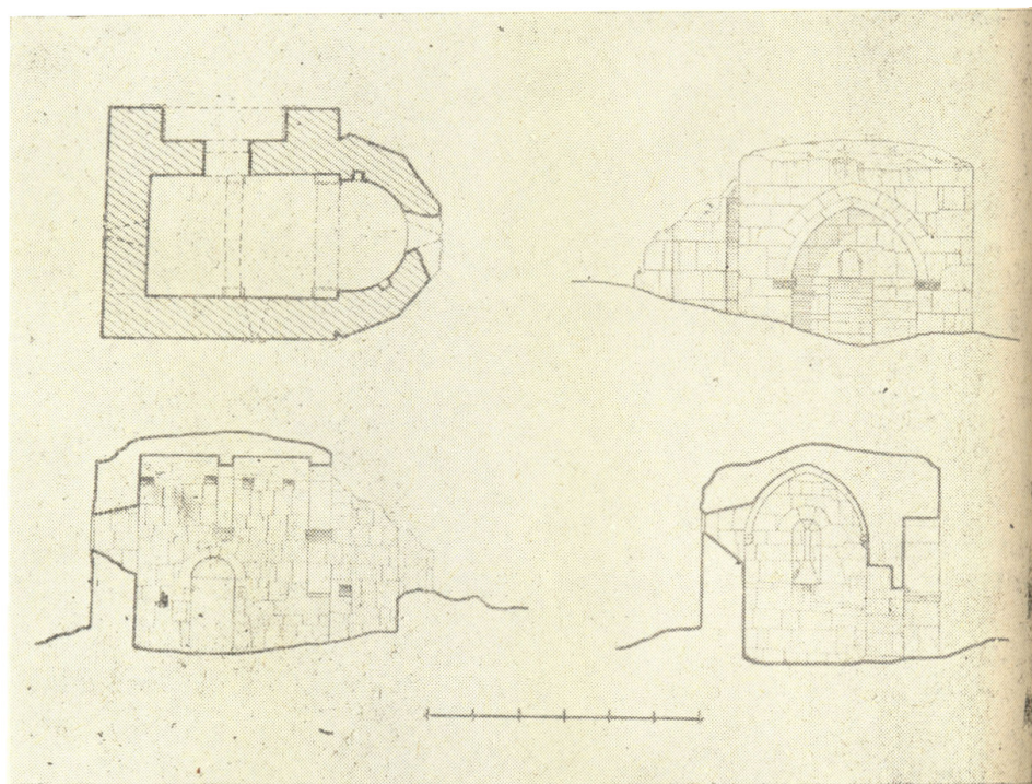
სურ. 1. გეგმა, გრძივი კრილი, ჩრდილოეთის ფასადი, განივი კრილი.
