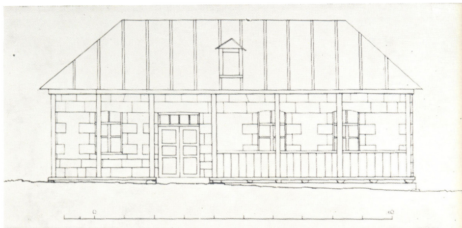
სურ. 2. ასპინძის რ-ნი, სოფ. სარო, ვასო თედორეს ძე ასპანიძის სახლის ფასადი.
