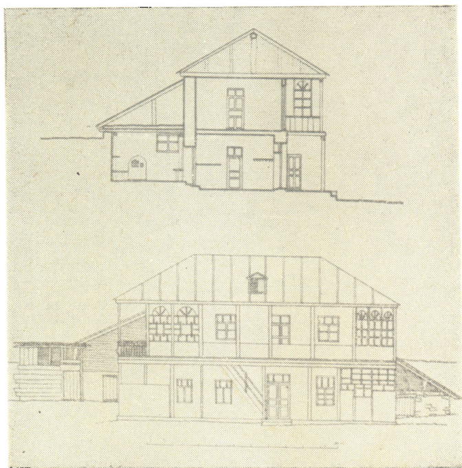
სურ. 2. ახალციხის რ-ნი. სოფ. ანდრიაწმინდა. შალვა გიორგის ძე ინასარიძის სახლის ფასალი და კრილი
