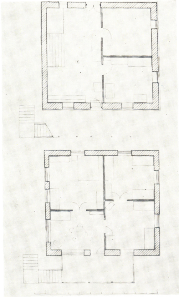
სურ. 1. ახალციხის რ-ნი. სოფ. ივლიტა. თამაზაშვილის სახლის გეგმები.
