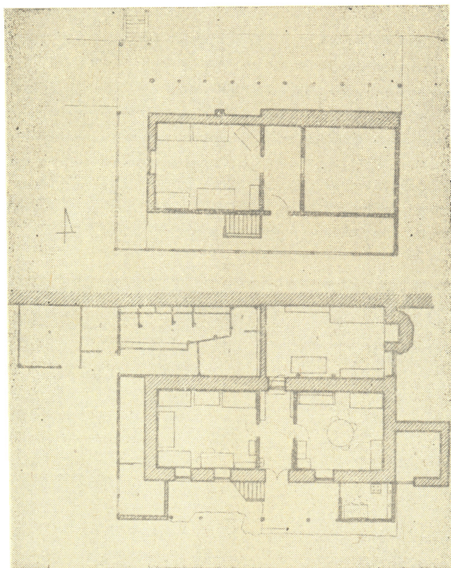
სურ. 1. ახალციხის რ-ნი, სოფ. ანდრიაწმინდა, შ. ინასარიძის სახლის გეგმები
