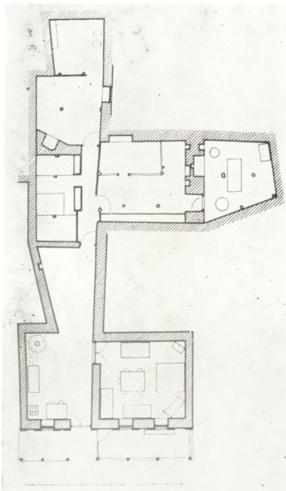
სურ. 1. ასპინძის რ-ნი, სოფ. სარო, ვასო თედორეს ძე ასპანიძის სახლის გეგმა.
