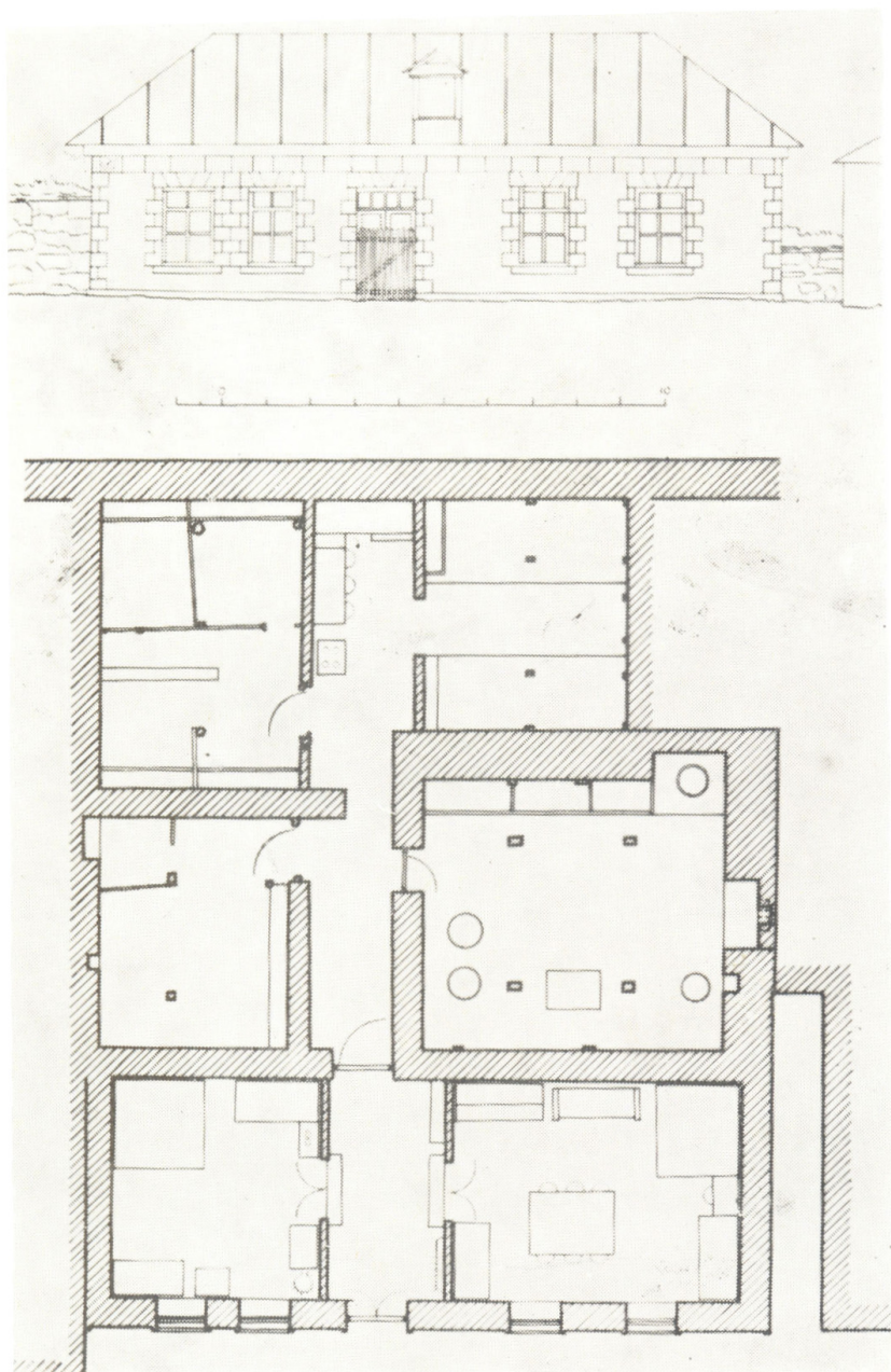
სურ. 1. ახალქალაქის რ-ნი, სოფ. გოგაშენი. ლადო ნათენაძის სახლის ფასადი და გეგმა.
