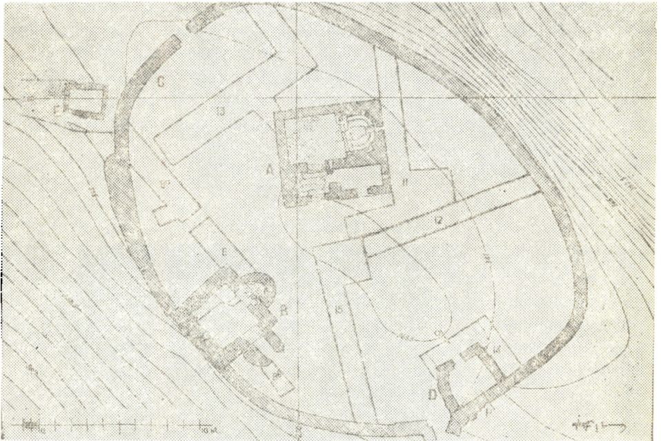
სურ. 2. სოფ. კუპრიაანთკარი. ქალეთის ხუროთმოძღვრული კომპლექსის გეგმა: A — წმ. გიორგის ეკლესია, B — კოშკი, C — გალავნი, D — ნაგებობის ნანგრევები, E — აკლამა, 8, 8 a , 8 b , 11, 12, 13, 14 და 15 — ზონდავები
