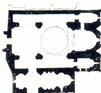
3. МЦХЕТА. Самтавро. План
