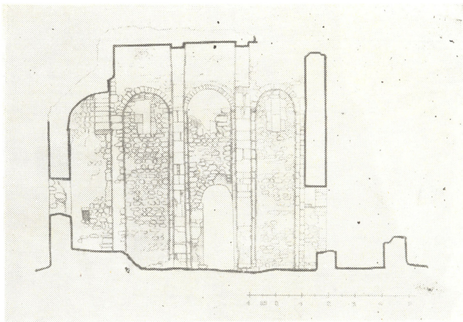
რუისპირის ვეელაწმინდის ეკლესიის გრძივი განაკვეთი
