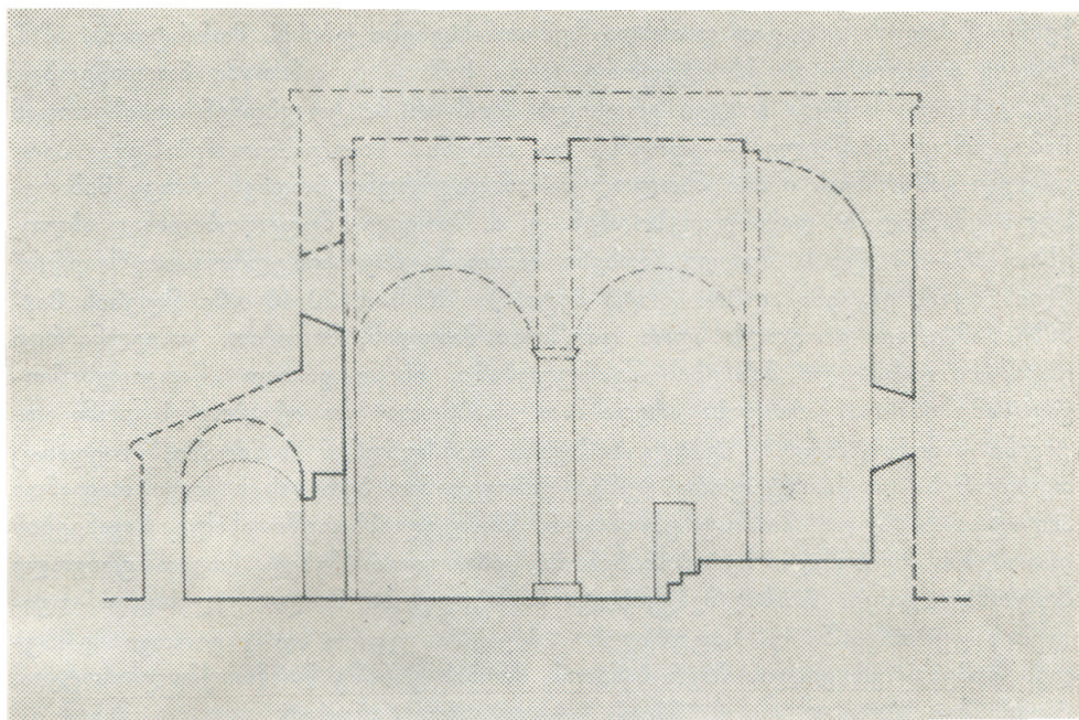
ფოთოლეთი. გრძივი კრილი. ხელი ჩრდილოეთისაკენ
