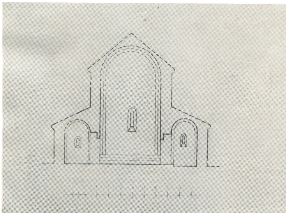
განივი კრილი. ხელი აღმოსავლეთისაკენ
