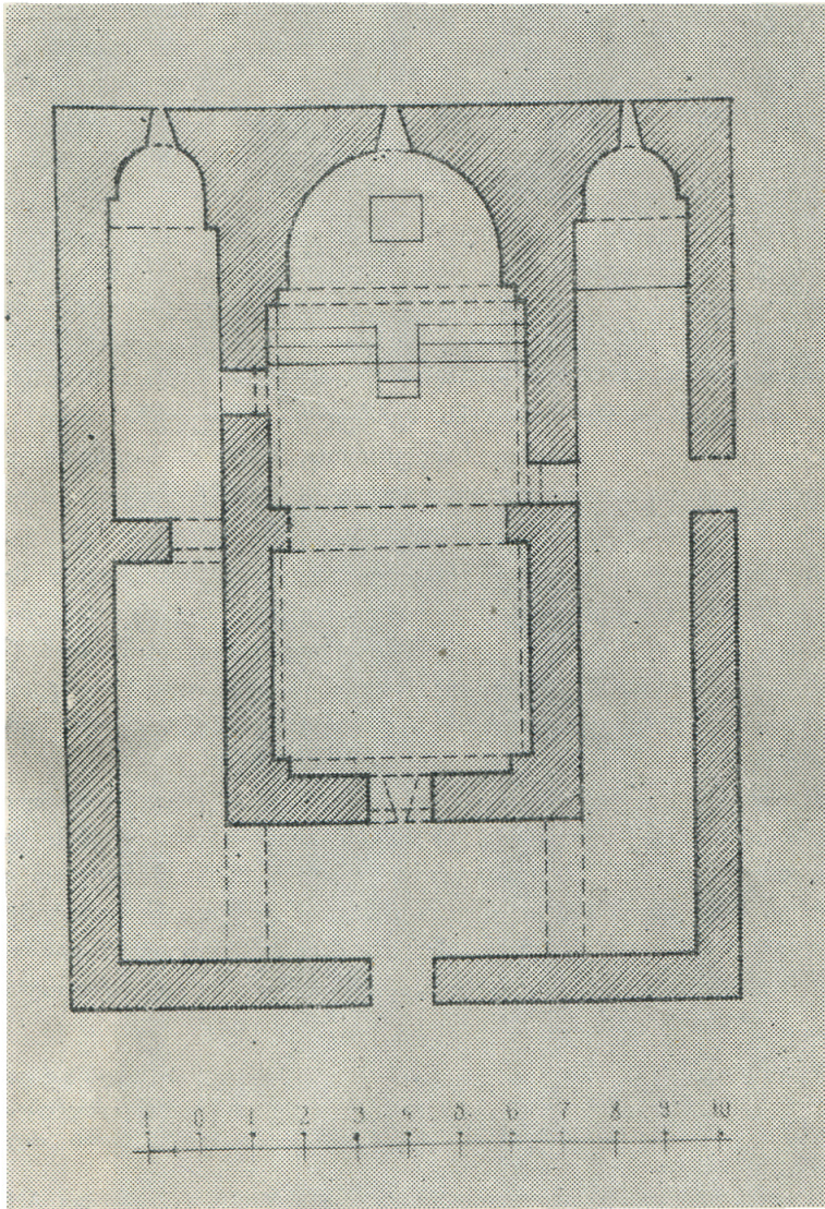
ფოთოლეთი. გეგმა
