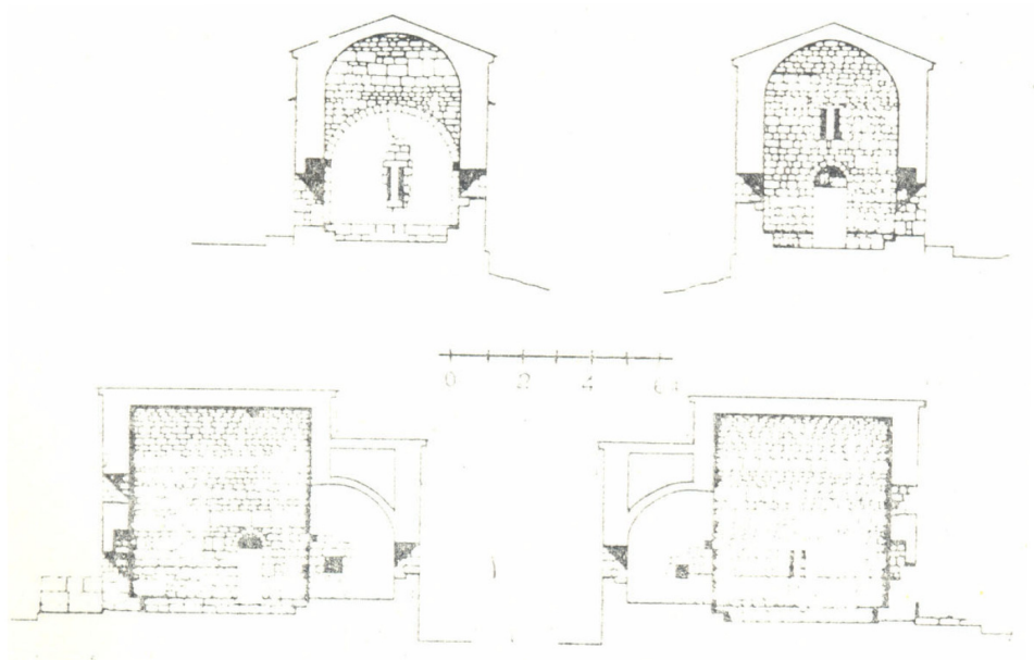
სურ. 2. ნოქალაქევი. ეკლესია „მისარონი“. განკვეთები
