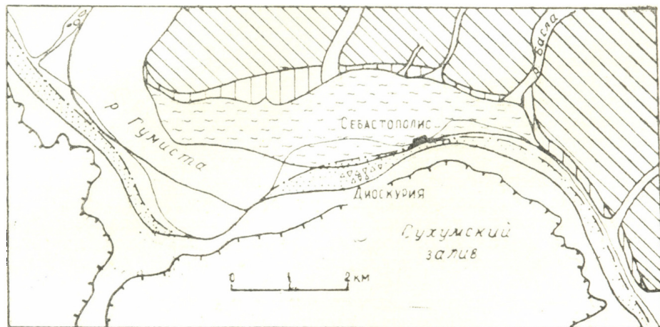
Рис. 3. Палеогеографическая схема развития Сухумского полуострова с V в. до н. э. по V в. н. э. (по И. П. Балабанову). Условные обозначения см. рис. 2.
