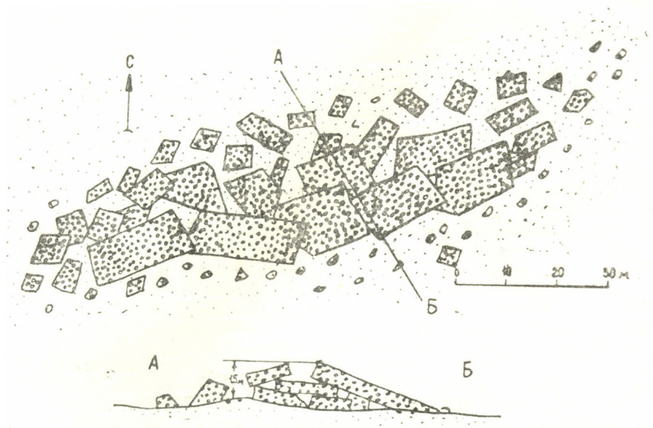
Рис. 4. Развал крепостных стен в районе створа 55, глубина моря 7 м (зарисовка И. Гусакова 20.10.1983 г.)
