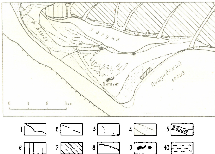
Рис. 2. Палеогеографическая схема развития Пицундского полуострова с V в. до н. э. по V в. н. э. (по Балабанову И. П. и др., 1981)
