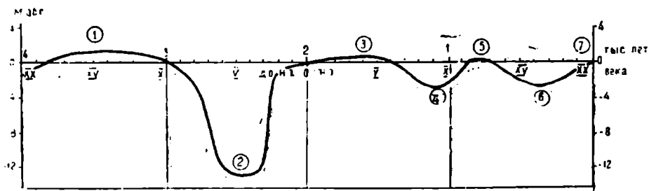
Рис. 1. Кривая колебания уровня Черного моря за последние 4 тыс. лет (по Балабанову И. П. и др., 1981). Трансгрессивные фазы: 1 — новочерноморская, 3 — шимфейская, 5 — средневековая, 7 — современная. Регрессивные фазы: 2 — фангорийская, 4 — раннесредневековая, 6 — позднесредневековая.
