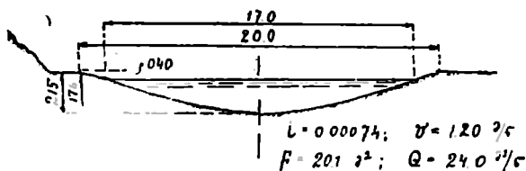
არხის კვეთი სტავესთან პიკ 0
