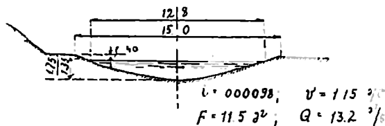
არხის კვეთი პიკ 814
