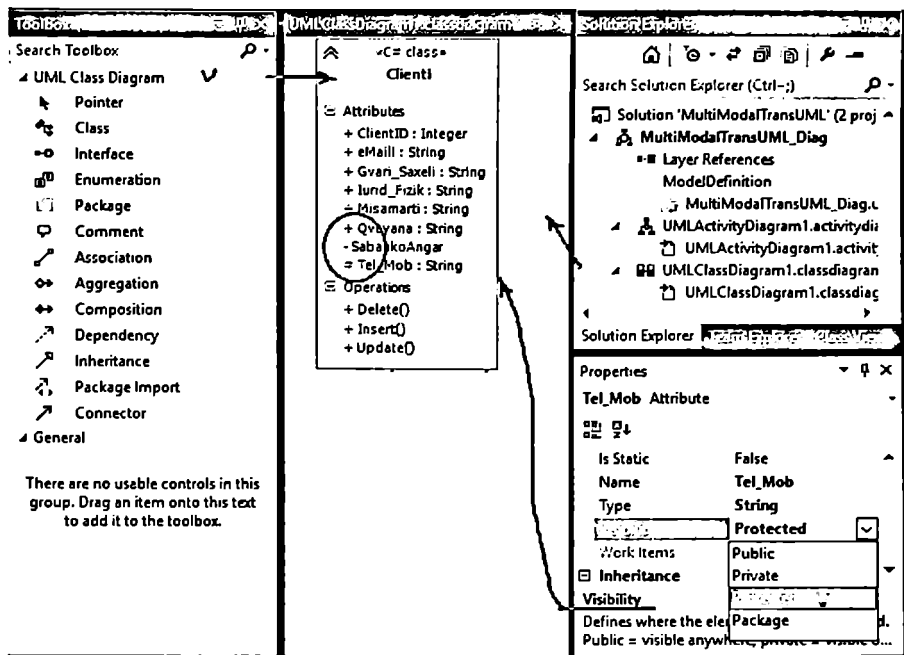
ნახ.3.1. კლასის ფორმირების მაგალითი VisualStudio.NET გარემოში
