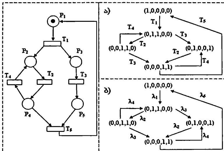
ნახ.4.3. სტოქასტური პეტრის ქსელი: ა) მიღწევად მარკირებათა „სიით“; ბ) ევოლუტორ მარკოვის ჯაჭვით
