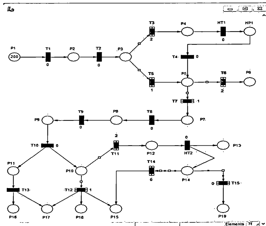
ნახ.4.9. იმიტაციური პროცესის დასაწყისი და კონფლიქტური კვანძთა ჯგუფები პეტრის ქსელის გრაფში (Visual Object Net++)
