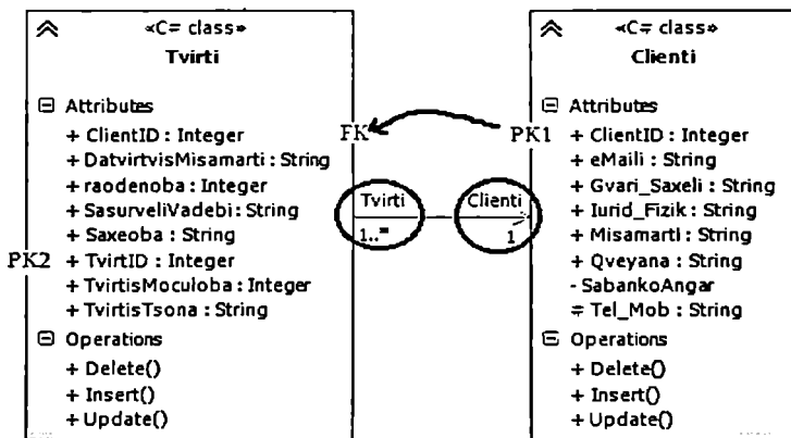
ნახ.3.2. კლასის დამატება დიაგრამაზე
