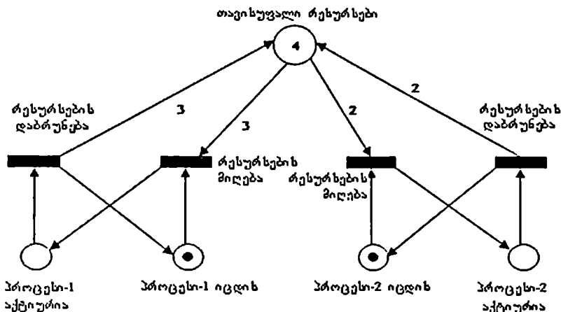
ნახ.4.2. კლასიკური პეტრის ქსელი „რესურსების განაწილების“ ამოცანა
