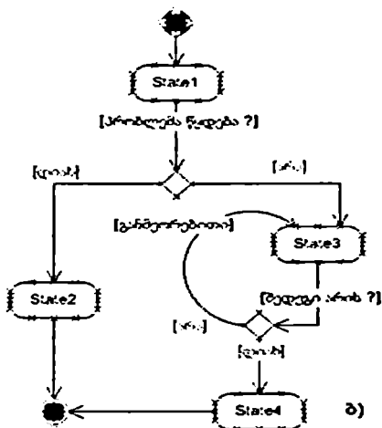
ნახ.3.13. Statechart-ის პანელი (ა) და მდგომარეობათა დიაგრამის ზოგადი მაგალითი
