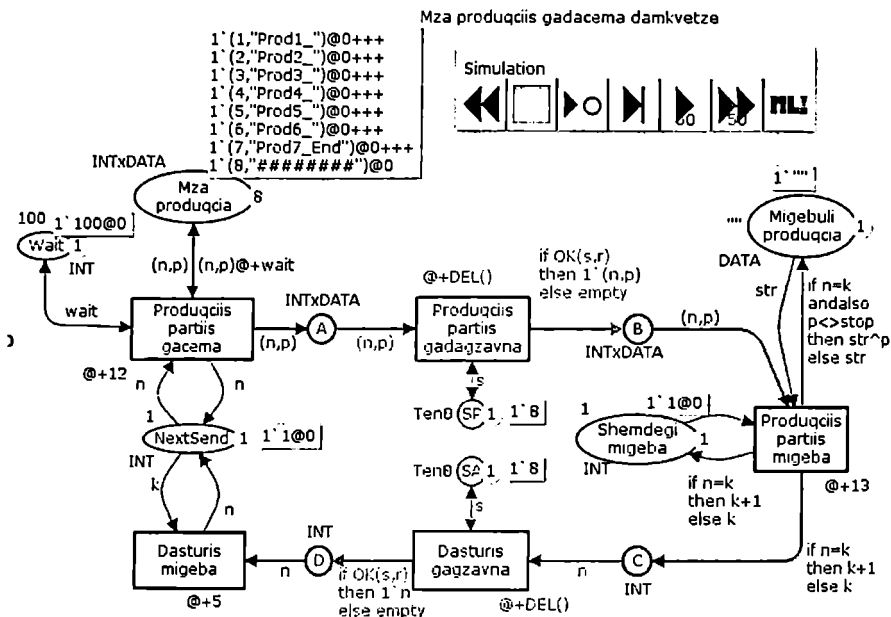
ნახ.4.12. იმიტაციური მოდელი CPN ქსელით „პროდუქციის მიწოდება“
