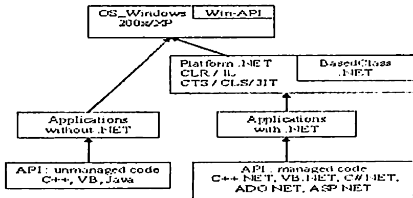
ნახ.1.10. .NET-ის კონცეფცია
