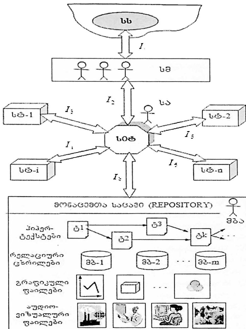
ნახ.1.9. ინტეგრირებული საინფორმაციო მართვის სისტემის გაშლილი სქემა
