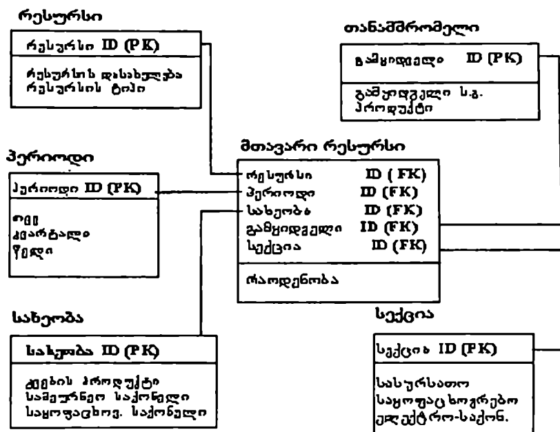
ნახ.2.1. რადიალური სქემა
