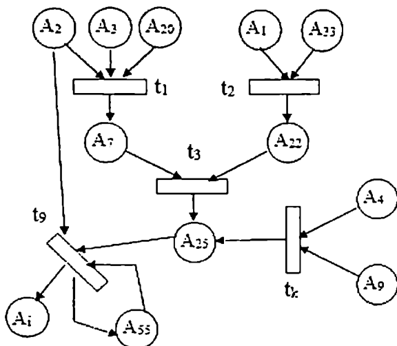
ნახ. 2.7. ატრიბუტების სქემის პეტრის ქსელის გრაფი
