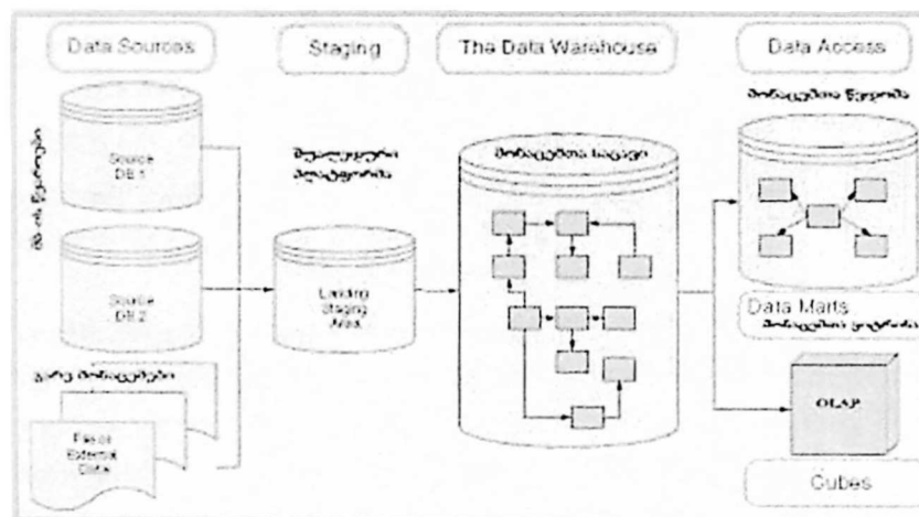
ნახ.1.4. ინმონის მონაცემთა საცავის მოდელი ერდნობოდა აღმავალ ტექნოლოგიას
