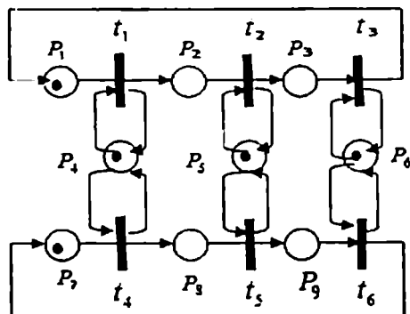
ნახ.5.5. პეტრის ქსელის გრაფი: S_1(P_1, P_2, P_3), S_2(P_7, P_8, P_9) - 2 სერვერი C(P_4, P_5, P_6) კლიენტი; P - პოზიცია (სერვერის მდგომარეობა); T - გადასასვლელი; მარკერი - შავი წერტილი; P_1 და P_7 - აქტიურებია; t_1 ან t_4 გაიხსნება P_4 -ის (მოთხოვნისა) მარკერით
