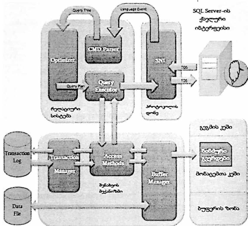
ნახ.4.5. SQL Server-ის არქიტექტურა [107]
