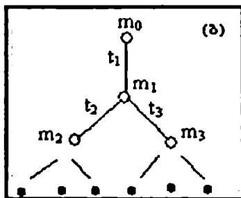
ნახ.5.10. პეტრის ქსელის (ნახ.5.9) შესაბამისი პროცესის გადასვლების მატრიცა (ა) და მიღწევადობის ხის ფრაგმენტი (ბ)
