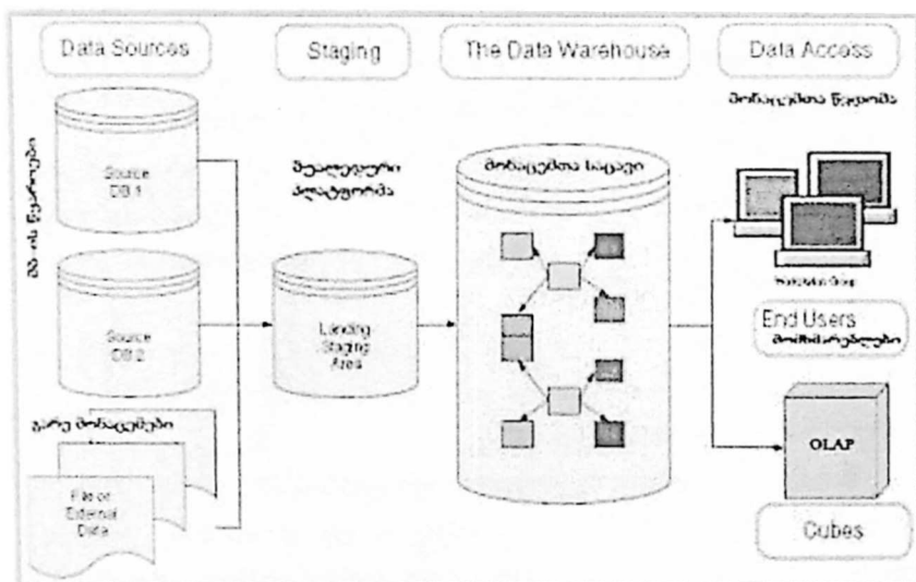
ნახ.1.5. კიბალის მონაცემთა სასიცოცხლო ციკლის მოდელი
