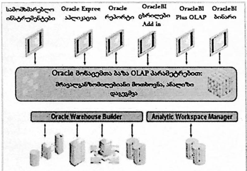
ნახ.5.20. Oracle OLAP -ის არქიტექტურა
