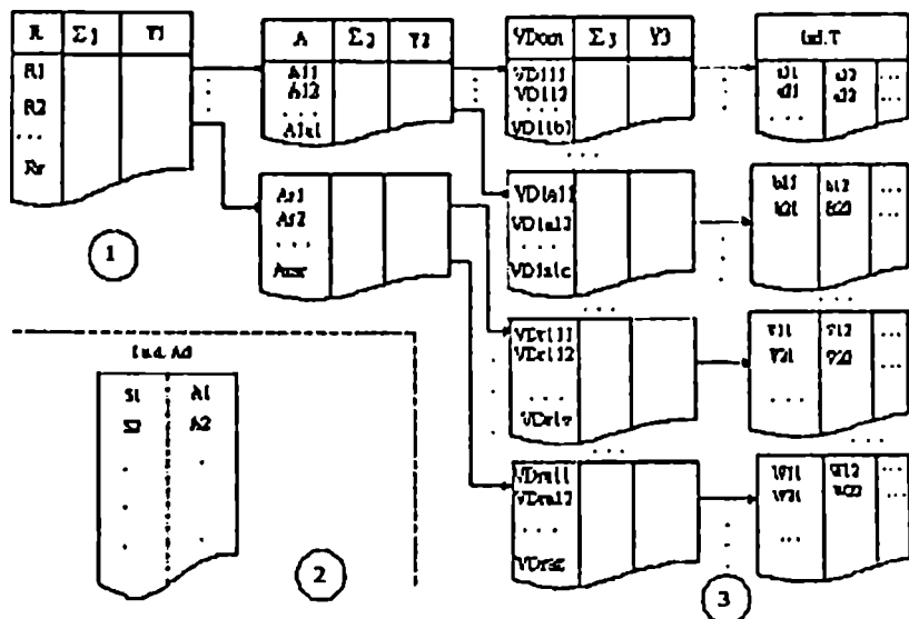
ნახ. 2.3. მეტაინფორმაცია - მართვის სამდონიანი კატალოგი
