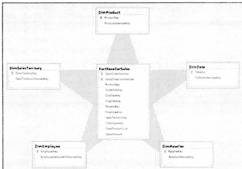
ნახ.1.2-ა. სქემა „ვარსკვლავი“
