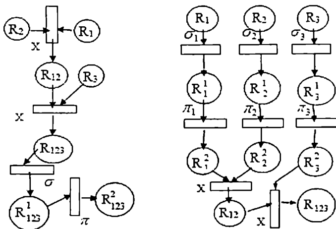
ნახ. 2.8. რელაგიათა სქემის პეტრის ქსელი გრაფი
