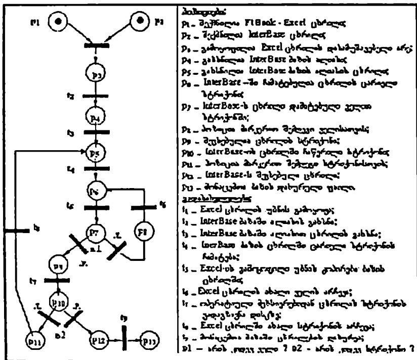
ნახ.2.9. პეტრის ქსელის გრაფიკული ლილაგისთვის ButtonClick - Import
