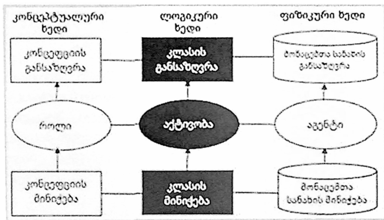
ნახ.1.7. მეტაპროცესის მოდელის სამი ხედი
