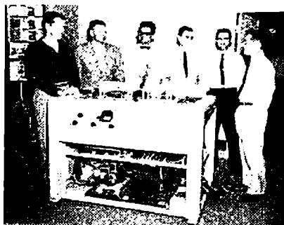
VRX-1000 - პირველი კომპერ- ციული ვიდეომაგნიტოფონი (1956), ფირმა „AMPEX“ ის ტექნიკური ჯგუფი
