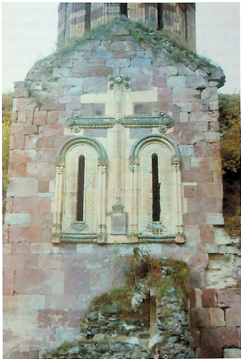
ჰუჯაბის მონასტრის მთავარი ტაძრის სამხრეთი ფასადი
