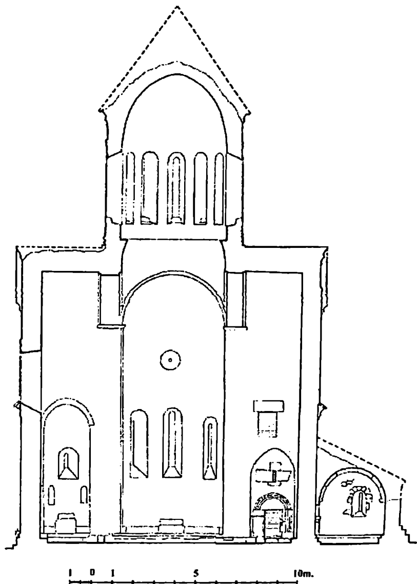
ჰუჯაბის ტაძრის სარესტავრაციო საპროექტო განაკვეთი აღმოსავლეთით შედგენილი აკაკი შავერდაშვილი მიერ
