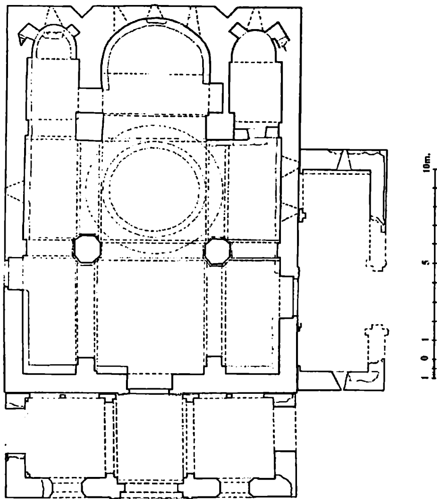
ჰუჯაბის მთავარი ტაძრის გეგმა შედგენილი აკაკი შავერდაშვილის მიერ
