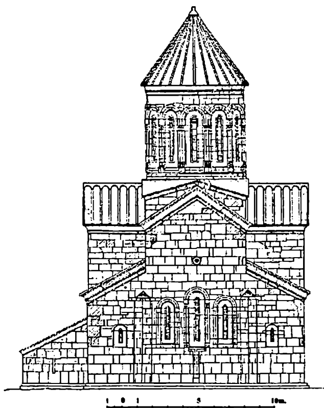
ჰუჯაბის მთავარი ტაძრის სარესტავრაციო პროექტი. პროექტის ავტორი არქიტექტორ-რესტავრატორი აკაკი შავერდაშვილი
