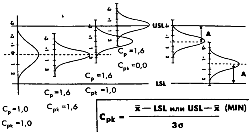
ნახ. 27 პროცესის აწყობის ინდექსი.
