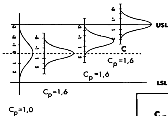
ნახ. 26. პროცესის შესაძლებლობის ინდექსი
