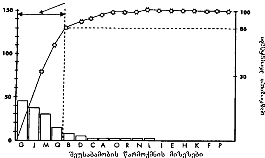
პირველი რიგის ზომების მიღების სფერო ნახ.22 პარეტოს დიაგრამა
