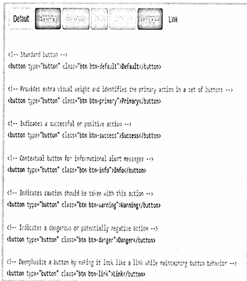
ნახ. 3. bootstrap ბიბლიოთეკის ფრაგმენტო
