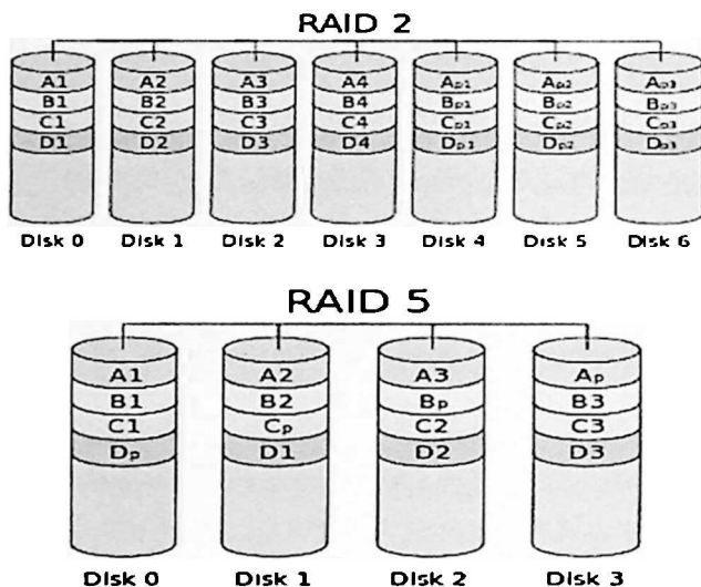
ნახ.2.6. დისკური მასივები RAID_2 და RAID_5
