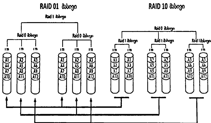
ნახ.2.7. დისკური მასივები RAID_01 და RAID_10
