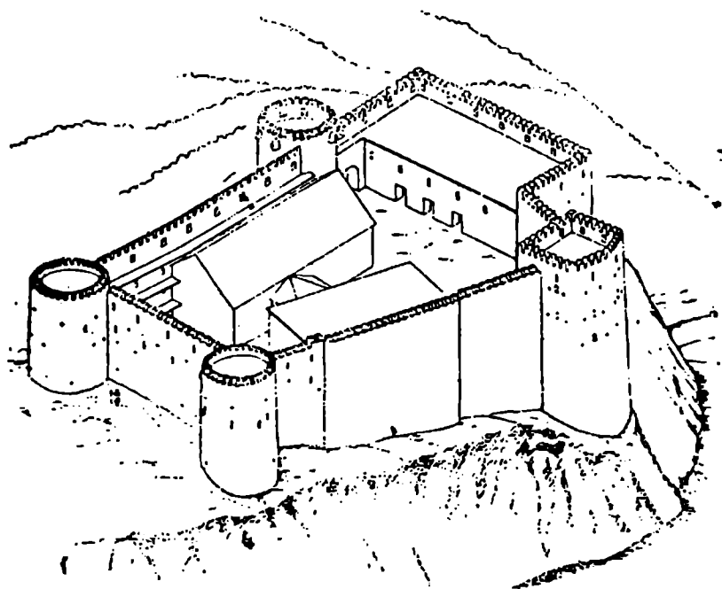
ბელოთის ციხე-სასახლე. რეკონსტრუქციის პროექტი.
