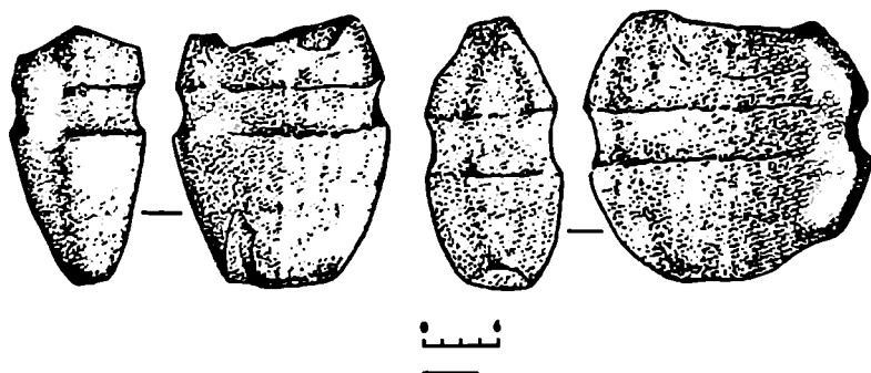
სურ. 4. უროების ტიპები ტვიბრაშერას გამონამუშევრებიდან (ჩართოლანი შ. 2010: 46)
