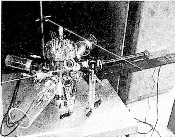
დოს ადამსონის ნაციონალური ღიაობის ექსპერიმენტული დანადგარი გაცივებული ჩაქვრული იონების ვაკუუმური სისტემა
