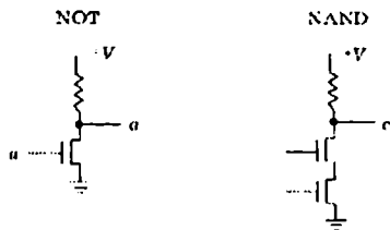
ნახ. 2. ტრანზისტორული წრედი NOT და AND-ისათვის
