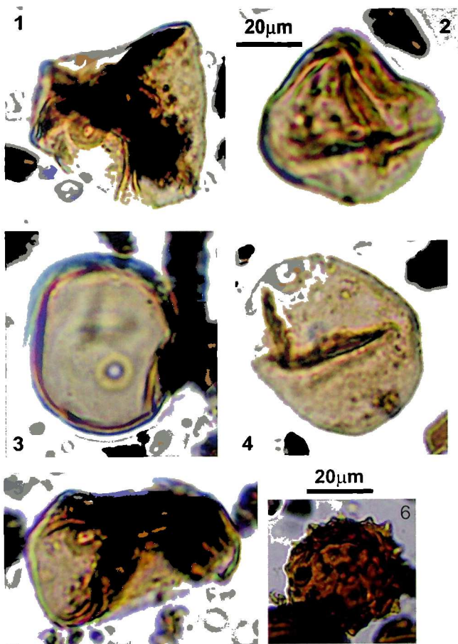
სურ. 45. ნამოსახლარი ნაცარგორა. ტრილ №2-ის კულტურულ ფენებში აღმოჩენილი სათესი მარცვლოვნებისა და მათი ხარველების მტვერი; 1,2,3 - ხორბალი ( Triticum ); 3,4 - განუსაზღვრელი სათესი მარცვლოვანი ( Cerealia ); 6 - ნარი ( Carduus ).
