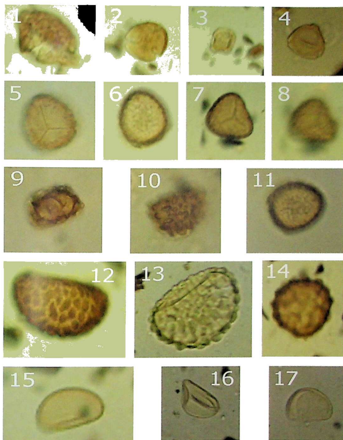
სურ. 7. თისელის სერის ნამოსახლარი. კულტურულ ფენებში აღმოჩენილ მცენარეთა მცენარე და გვიმრების სპორები: 1, 2 - მუხა ( Quercus ); 3 - მურყანი ( Alnus ); 4 - თხილი ( Corylus ); 5-8 - ქვრის გვიმრა ( Pteridium ); 9 - ჩადუნა ( Dryopteris ); 10 - გვიმრუკა ( Asplenium ); 11 - გვიმრანაირები (Polypodiaceae); 12,13 - კილაპურა ( Polypodium vulgare ); 14 - გველის ენა ( Ophioglossum ); 15 - განუსაზღვრელი გვიმრანაირები (Undiff. Polypodiaceae)
