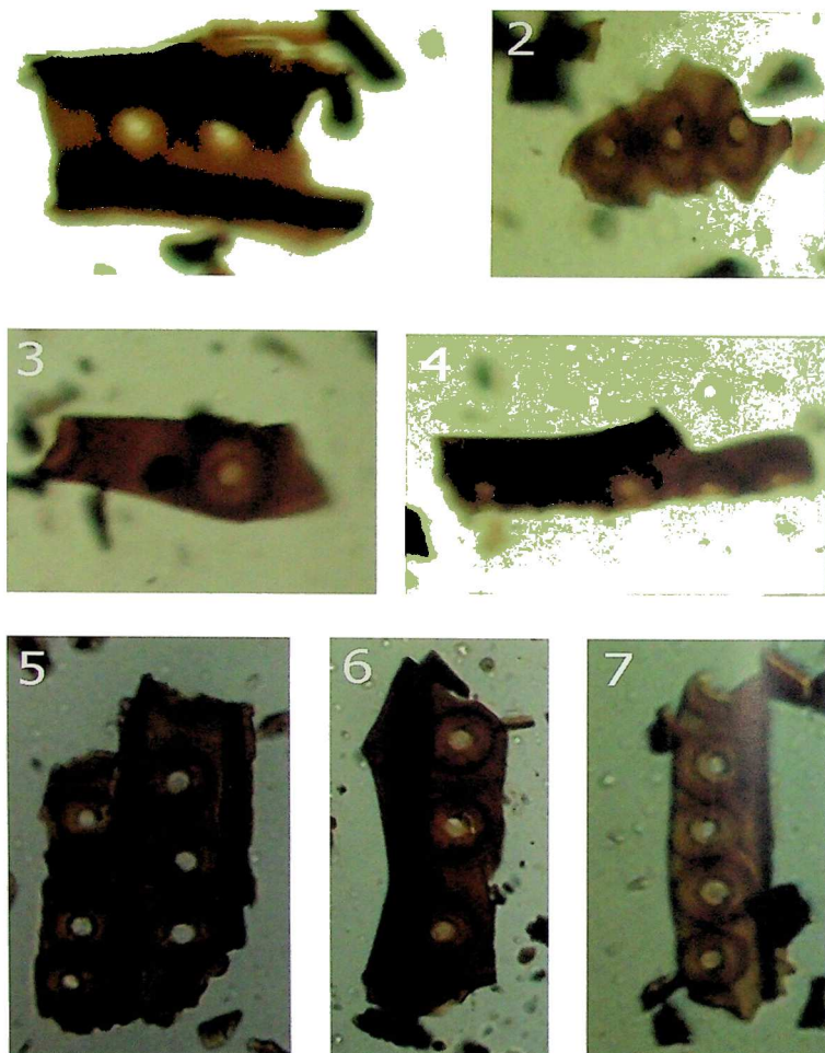
სურ. 4. თიხელის სერის ნამოსახლარი. ცულის ტარში აღმოჩენილი ფიჭვის მერქნის ტრაქეალური უჯრედები.
