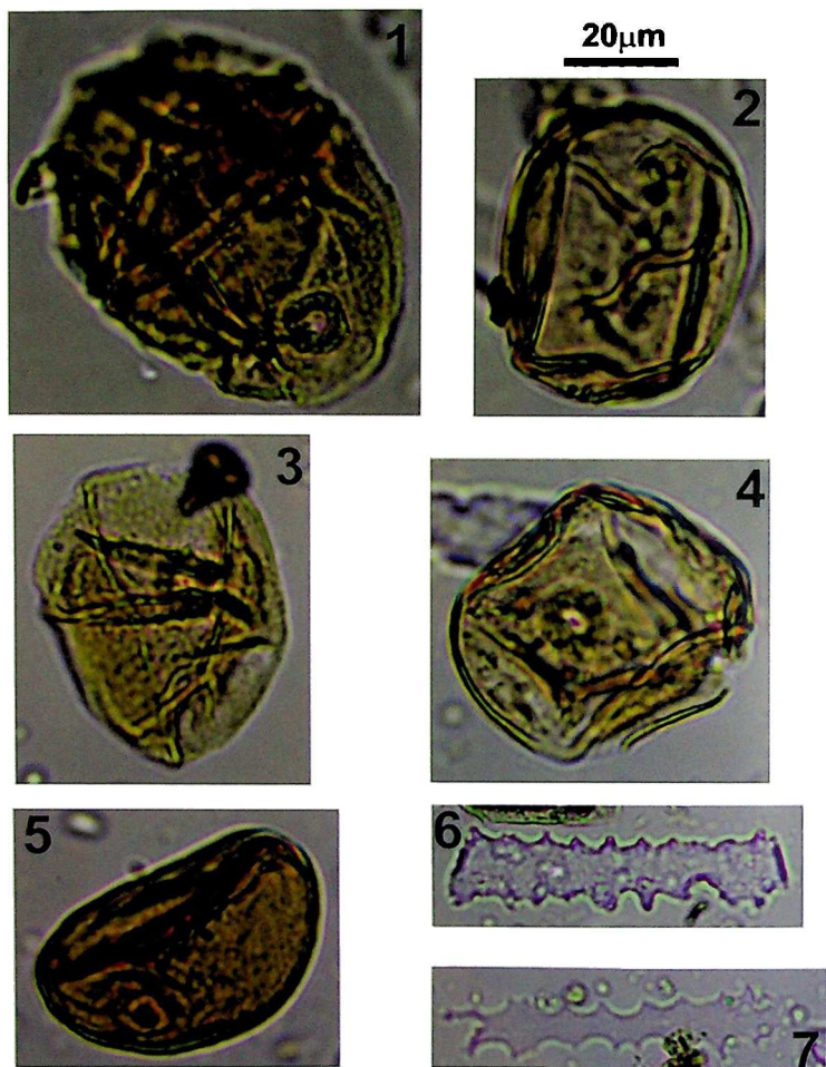
სურ.14. ჭობარეთი. სამეურნეო ორმოებიდან მოპოვებულ ორგანულ ნაშთებში აღმოჩენილი ხორბლის მტკერი (1-5) და ხორბლის ფიტოლიტები (6,7).
