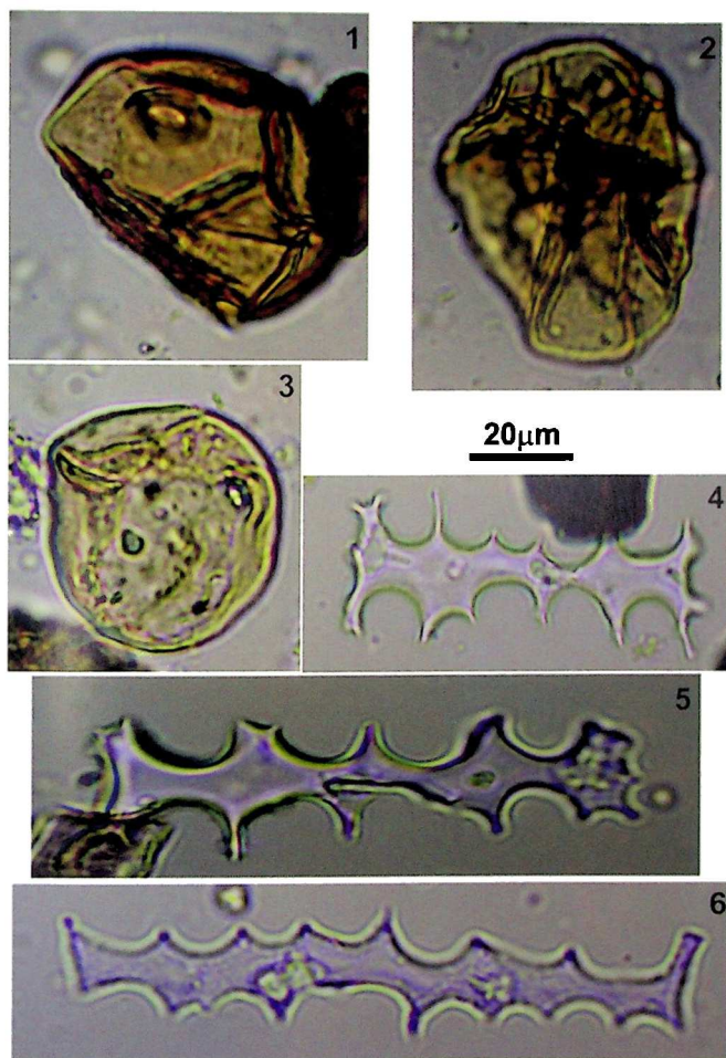
სურ. 15. ჭობარეთი. სამეურნეო ორმოებიდან მოპოვებულ ორგანულ ნაშთებში აღმოჩენილი ხორბლის მტვერი (1,2), განუსაზღვრელი სათესი მარცვლოვნის მტვერი (3) და ხორბლის ფიტოლითები (4,5,6).
