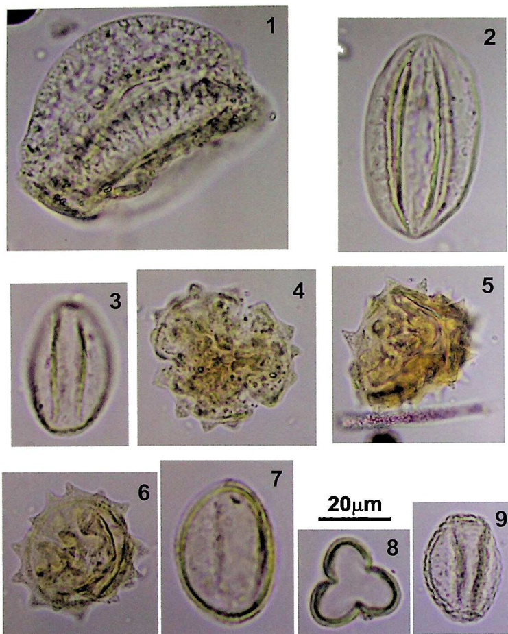
სურ. 65. თოფიოლას ყორღანი. იატაკის ფენაში აღმოჩენილ მცენარეთა მტკვერი: 1 - ფიჭვი ( Pinus ); 2 - ჭორის ძუა ( Ephedra ); 3 - მუხა ( Quercus ); 4,5,6 - წარშავი ( Carduus ); 7,8 - მატიტელა ( Polygonum ); 9 - ზაია ( Ranunculus ).
