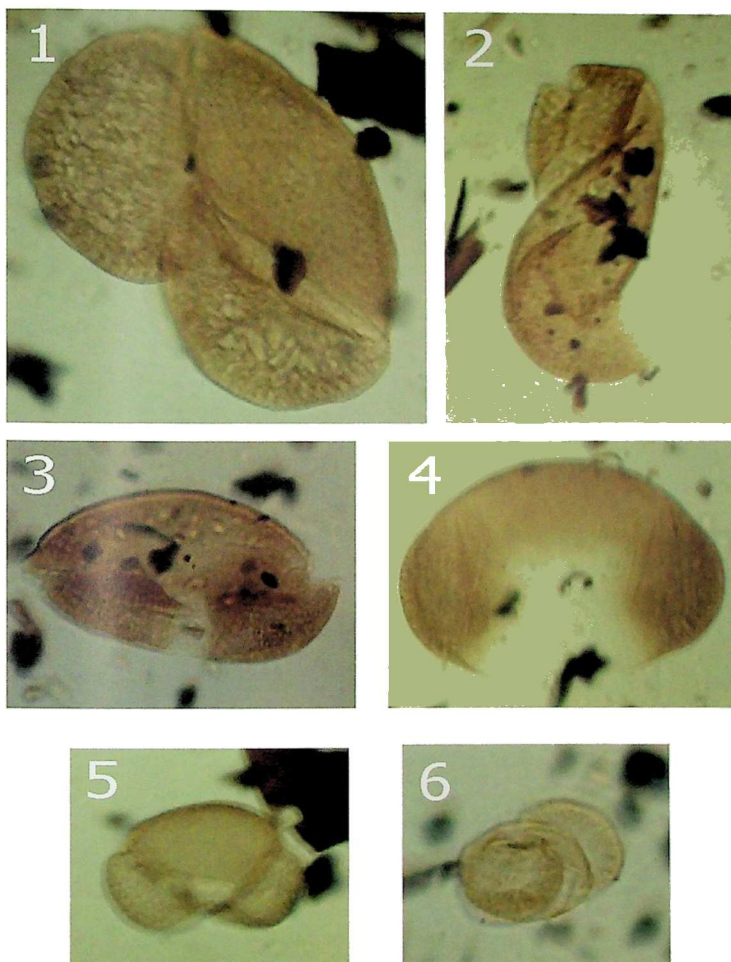
სურ. 5. თისელის სერის ნამოსახლარი. ცულის ტარში აღმოჩენილი წიწვოვნების მტერის მარცვლები: 1 - სოჭი ( Abies ); 2,3,4 - ნაძვი ( Picea ); 5,6 - ფიჭვი ( Pinus ).
