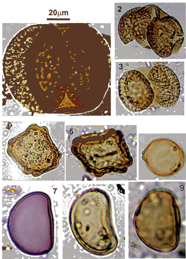
სურ. 39. ნამოსახლარი ნაცარგორა. ტრილ №1-ის კულტურულ ფენებში აღმოჩენილ მცენარეთა მცვერი და სპორები: 1 – სოჭი ( Abies nordmanniana ); 2,3 - ფიჭვი ( Pinus ); 4,5 - ძელქვა ( Zelkova carpinifolia ); 6 - ჯაგრცხილა ( Carpinus orientalis ); 7,8,9 - გვიმრების სპორები (Polypodiaceae).
