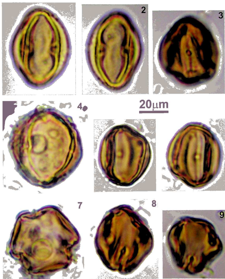
სურ. 50. ნამოსახლარი არადეთის ორგორა. ზოომორფული ჭურჭლის შიგთავსში აღმოჩენილი ჩვეულებრივი ვაზის მტერის მარცვლები.
