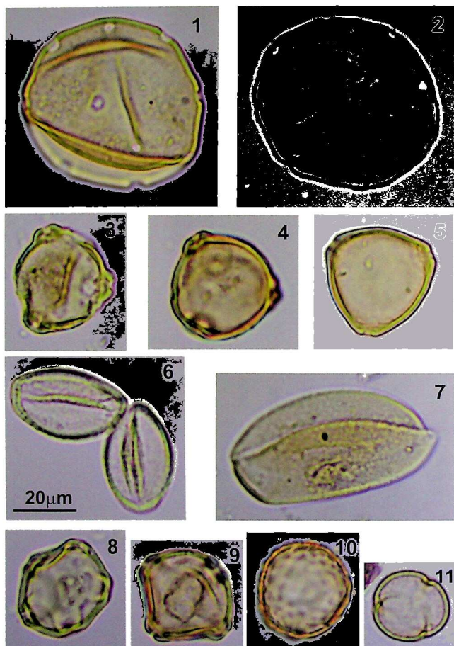
სურ. 28. დიდი ზომის ხელსაფეკვიდან მოპოვებულ ორგანულ ნაშთებში აღმოჩენილ მცენარეთა მტკვერი: 1, 2 - კაკალი ( Juglans regia ); 3, 4 - არეი ( Betula ); 5 - თხილი ( Corylus ); 6 - ტირილი ( Salix ); 7 - შროშანასებრნი ( Liliaceae ); 8, 9 - მურყანი ( Alnus ); 10 - შრაღალბარღა ( Plantago ); 11 - მუგუნა ( Rumex ).
