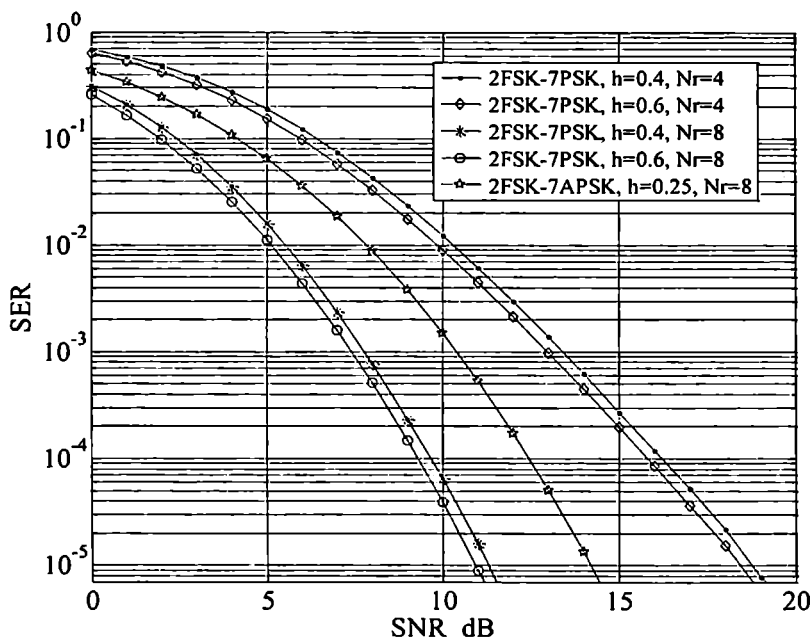
ნახ. 4.13. GSM სისტემის SER მახასიათებლები, როცა N_t = 4 რელეის არხისა და მკომბინირების MRC სქემისათვის
