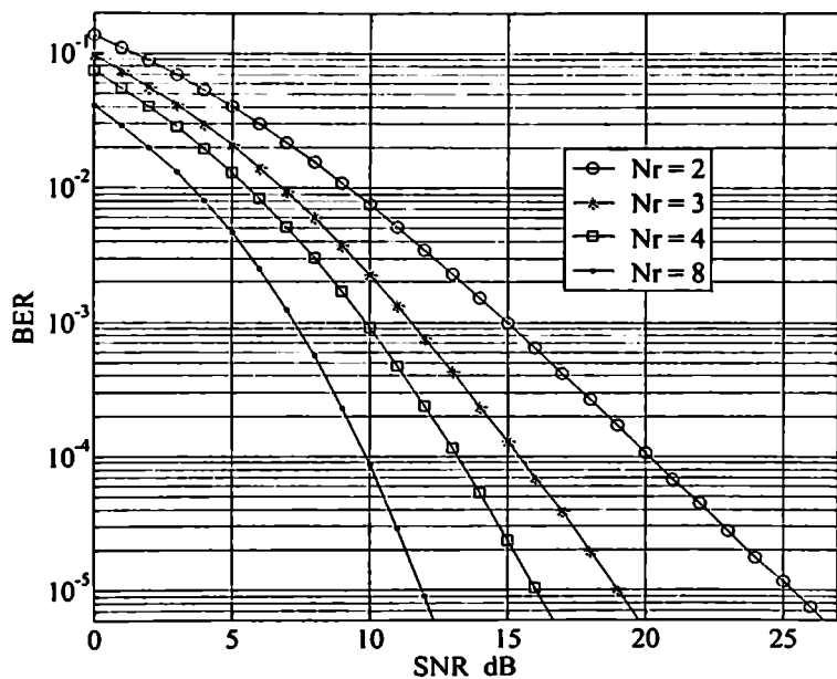
ნახ 4.8. MIMO-SM სისტემის BER მახასიათებლები, როცა a=1 , M=8 , N_t=2 , m=1 , S_E=4
