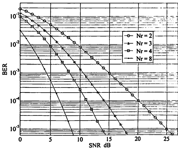
ნახ 4.7. MIMO-SM სისტემის BER მახასიათებლები, როცა a=1 , M=4 , N_t=4 , m=1 , S_E=4
