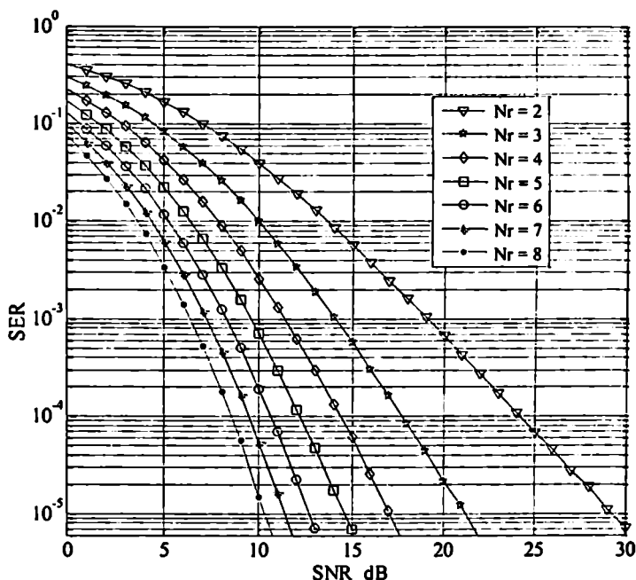
ნახ. 3.8. 2FSK-8PSK სიგნალის SER მაჩასიათებლები რელეის არხში კომბინირების MRC სქემის გამოყენებისას, როცა h=0.4
