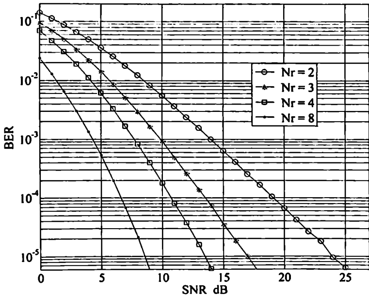
ნახ 4.6. MIMO-SM სისტემის BER მახასიათებლები, როცა a=1 , M=4 , N_t=2 , m=1 , S_E=3
