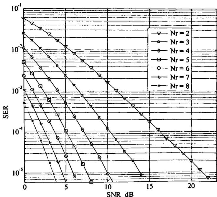
ნახ. 3.11. BPSK სიგნალის SER (BER) მაჩვენებლები რელის არხში, კომბინირების MRC სქემის გამოყენებისას
