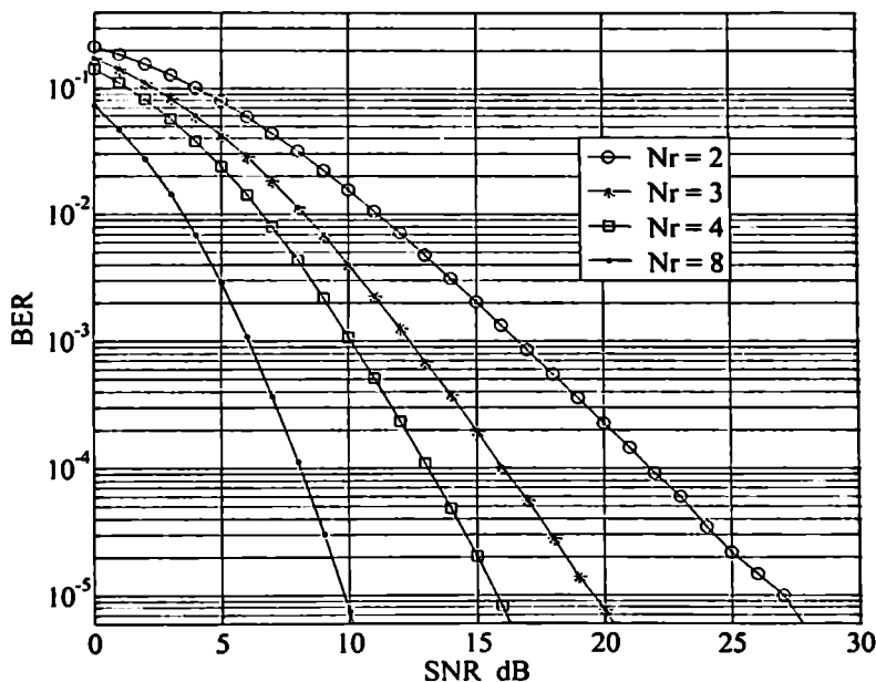
ნახ 4.4. MIMO-SM სისტემის BER მახასიათებლები, როცა a=1 , M=2 , N_r=2 , m=1 , S_E=2
