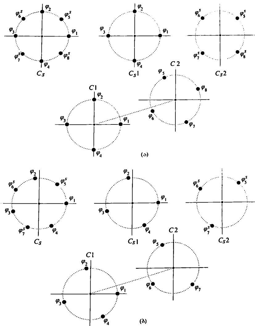
ნახ. 2.8. 2FSK-8PSK (ა) და 2FSK-7PSK (ბ) სიხნალოთა აგების პროცედურები
