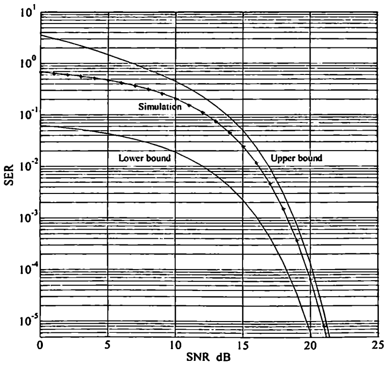
ნახ. 2.4. SER , ზედა საზღვარი (Upper bound), მოდელირებით მიღებული (Simulation) და ქვედა საზღვარი (Lower bound), 2D 11PSK სიგნალისათვის გაუსის არხში
