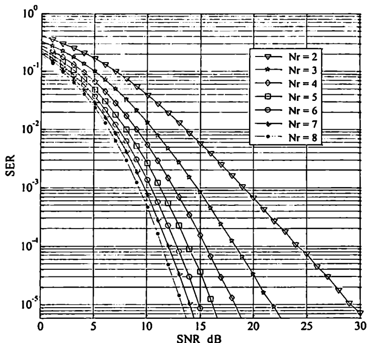
ნახ. 3.15. 2FSK-8PSK ( h=0.4 ) სისტემის SER მახასიათებლები PMRC სქემისათვის რელის არხში
