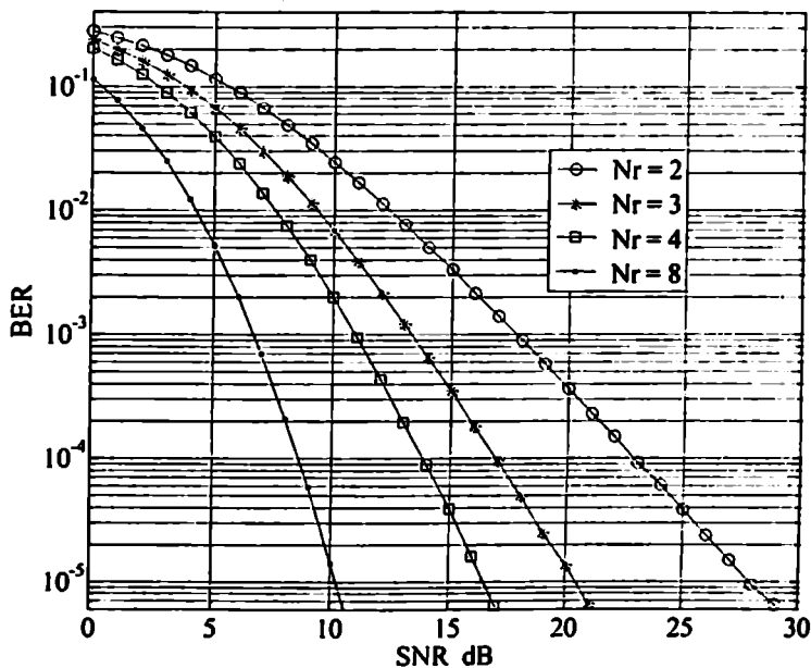
ნახ 4.5. MIMO-SM სისტემის BER მახასიათებლები, როცა a=1 , M=2 , N_r=4 , m=1 , S_E=3
