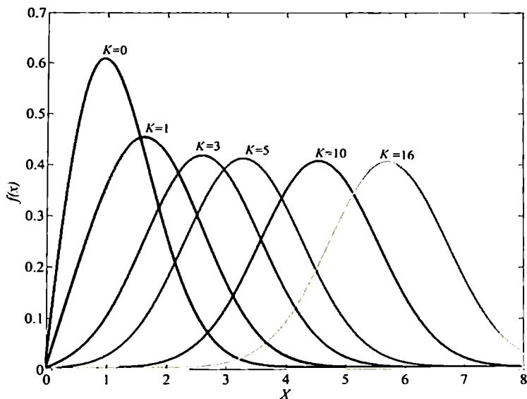
ნახ. 15. რაიის ალბათობის განაწილების სიმკვრივები
