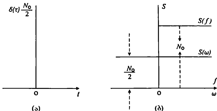
ნახ. 1.1. თეთრი ხმაურის კორელაციური ფუნქცია (ა) და სპექტრული სიმკერძე (ბ)
