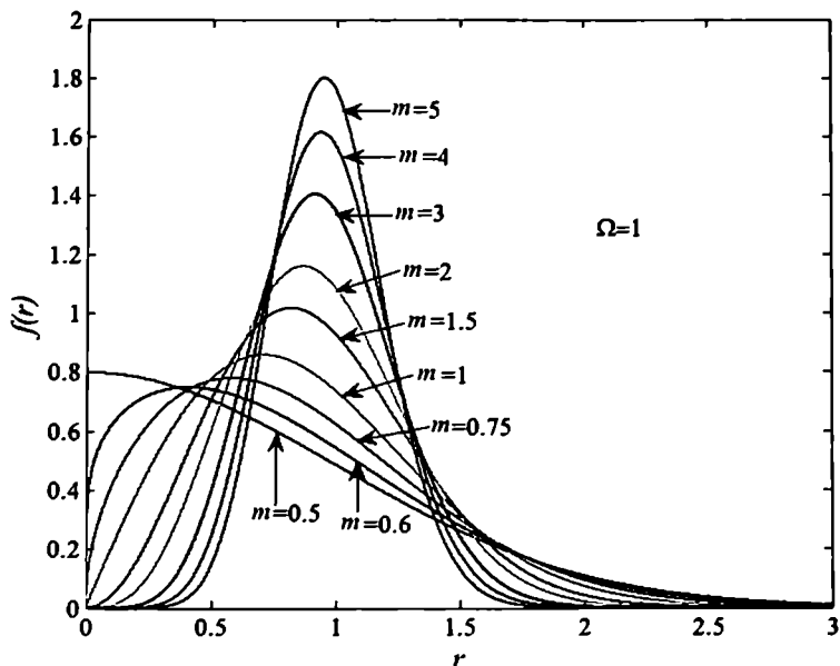
ნახ. 1.7. ნაკაგამის აღბათობის განაწილების სიმკვრივეები
