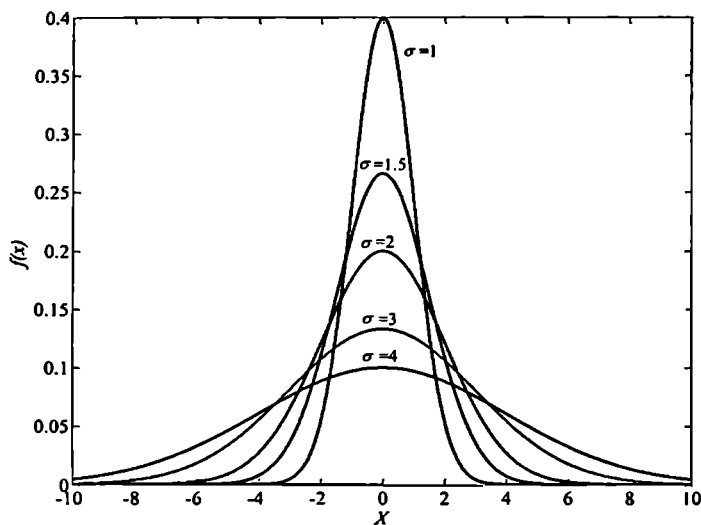
ნახ. 12. გაუსის ალბათობის განაწილების სიმკვრივეები
