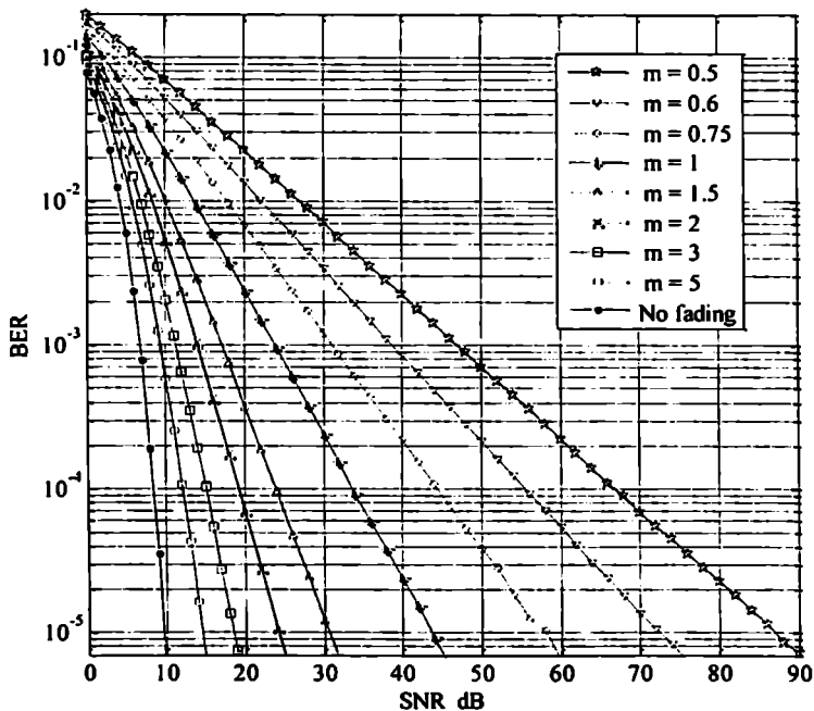
ნახ. 3.1. ბიტის შეცდომის ალბათობათა მახასიათებლები BPSK-თვის ნაკავამის არხში
