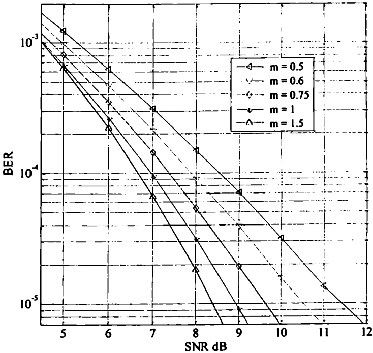
ნახ. 3.3. ბიტის შეცდომის აღბათობათა მახასიათებლები BPSK-თვის ნაკაგამის არხში, მიმღებ ანტენათა მიმორიგებით, როცა N_r = 8
