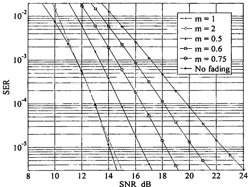
ნახ 4.12. GSM სისტემის SER მახასიათებლები, როცა M = 7 , N_t = 4 და N_r = 8 ნაკავშირის არხისა და კომბინირების SC სქემისათვის
