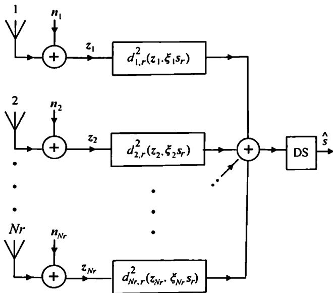
ნახ. 3.10. მაქსიმალური თანაფარდობის კომბინირების მოდერნიზებული სქემა
