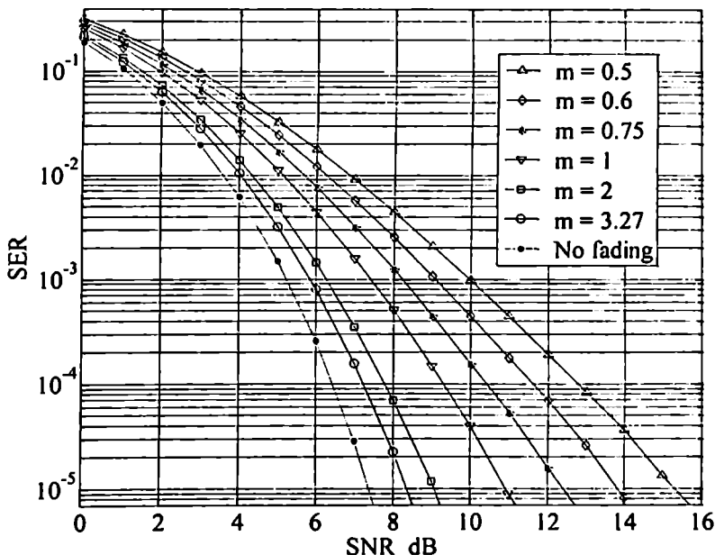
ნახ 4.14. GSM სისტემის SER მახასიათებლები, როცა M = 7 , h = 0.6 , N_f = 4 , N_r = 8 ნაკადების არხისა და კომბინირების MRC სქემისათვის
