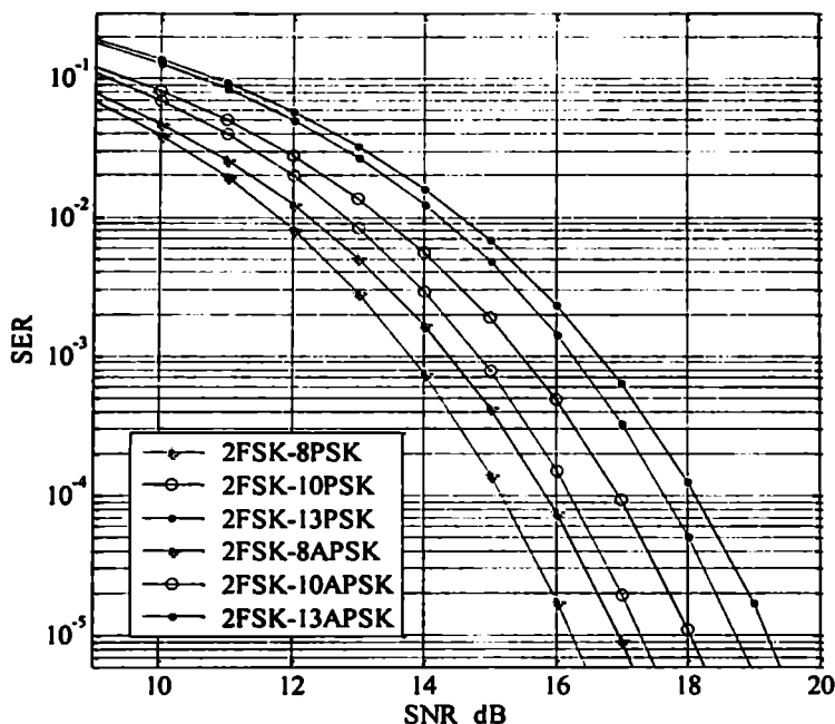
ნახ.2.14. ზოგიერთი 4D სიგნალის SER მახასიათებლები გაუსის არხში
