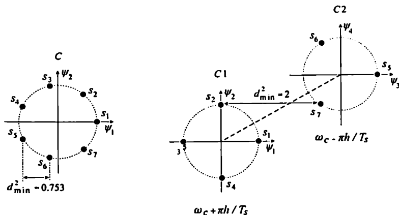
ნახ. 2.7. ჩვეულებრივი 2D 7PSK და 4D 2FSK-7PSK სიგნალთა ინტერპრეტაცია
