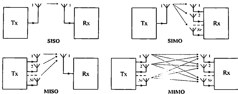
ნახ. 4.1. მიმღებ-გადამცემ ანტენათა შესაძლო კონფიგურაციები
