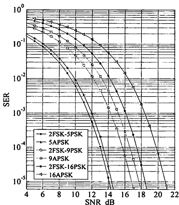
ნახ. 29. ზოგიერთი 2FSK-MPSK და MAPSK სიგნალის SER მახასიათებელი გაუსის არხისთვის, როცა h = 0.4
