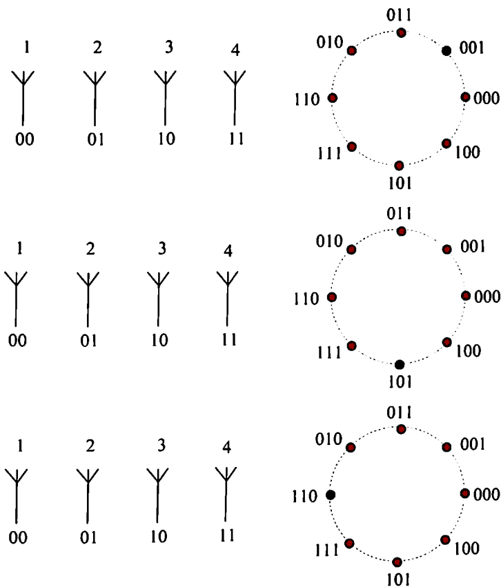
ნახ. 4.3. SM პროცესის ინტერპრეტაციის მაგალითი
