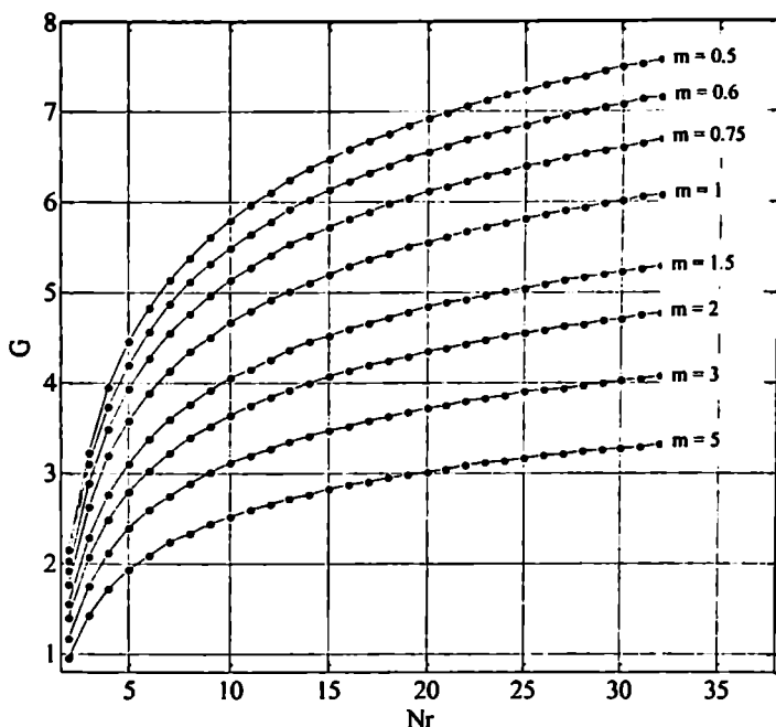
ნახ. 3.12. მიმორიგების ეფექტურობის შეფასება ნაკადის ფელინგის შემთხვევაში კომბინირების SC სქემისათვის
