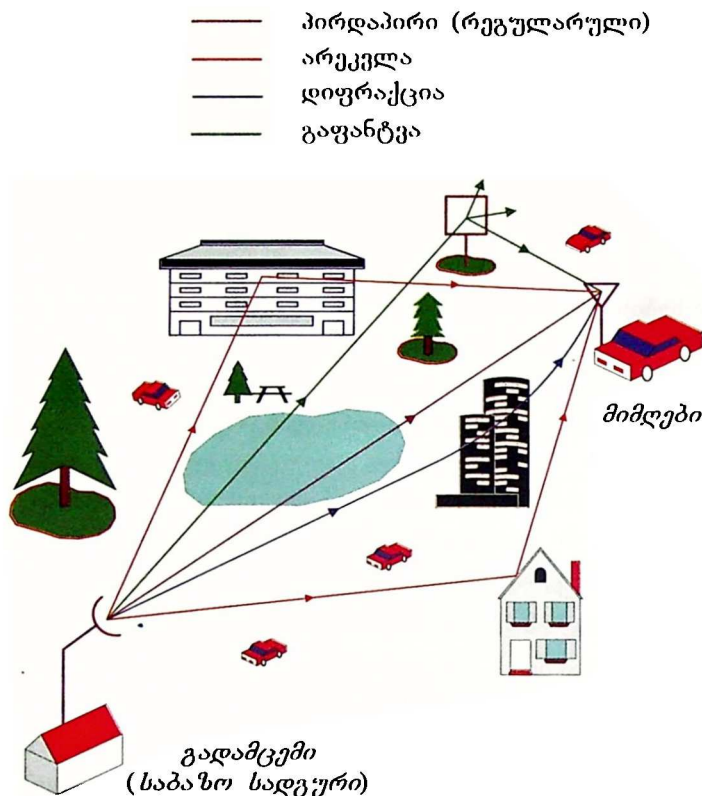
ნახ. 14. რადიოტალღების მრავალსიხივად გავრცელების სურათი
