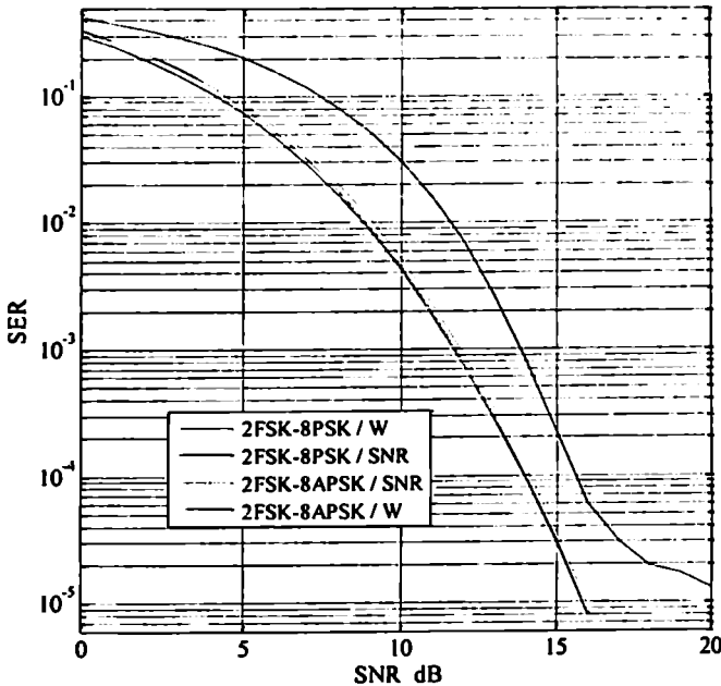
ნახ. 3.6. 2FSK-8PSK და 2FSK-8APSK სიგნალების SER მახასიათებლები რელეის არხში, კომბინირების SC სქემის გამოყენებისას, როცა N_r = 8
