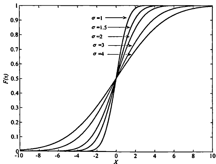
ნახ. 13. გაუსის ალბათობის განაწილების ინტეგრალური ფუნქციები
