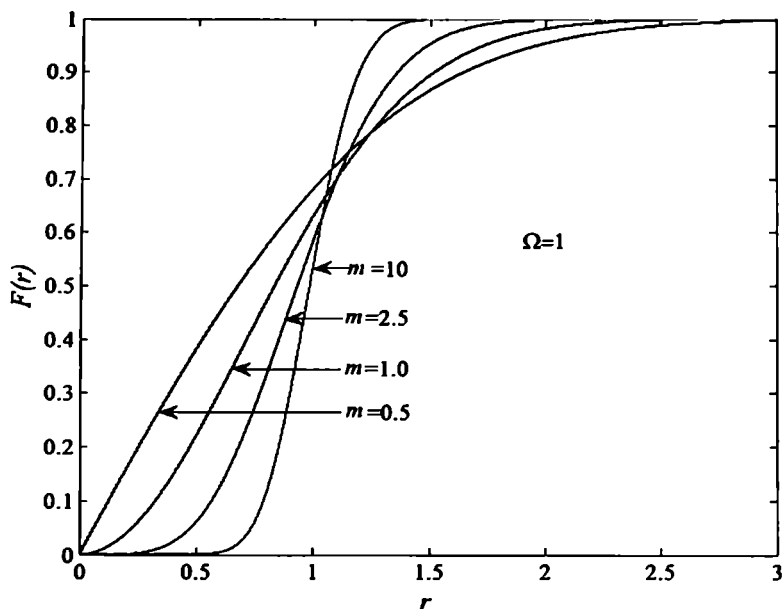
ნახ. 1.8. ნაკაგამის ალბათობის განაწილების ინტეგრალური ფუნქციები
