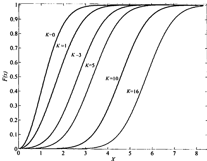
ნახ. 1.6. რაისის ალბათობის განაწილების ინტეგრალური ფუნქციები
