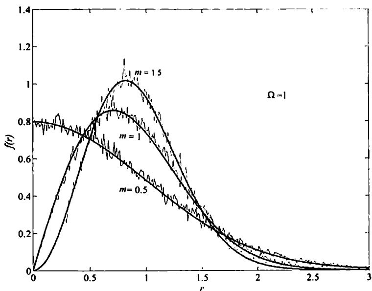
ნახ. 1.9. ნაკაგამის განაწილების სიმკვრივის მრუდები, მოდელირებით და ფორმულით
