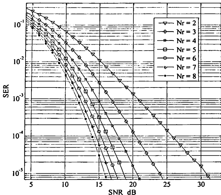
ნახ.3.5. 2FSK-8PSK სიგნალის SER მახასიათებლები რელეის არხში კომბინირების SC სქემის გამოყენებისას, როცა h=0.4
