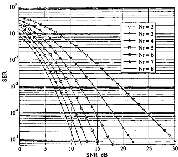
ნახ. 3.9. 2FSK-8APSK სიგნალის SER მახასიათებლები რელეის არხში კომბინირების MRC სქემის გამოყენებისას, როცა h = 0.3
