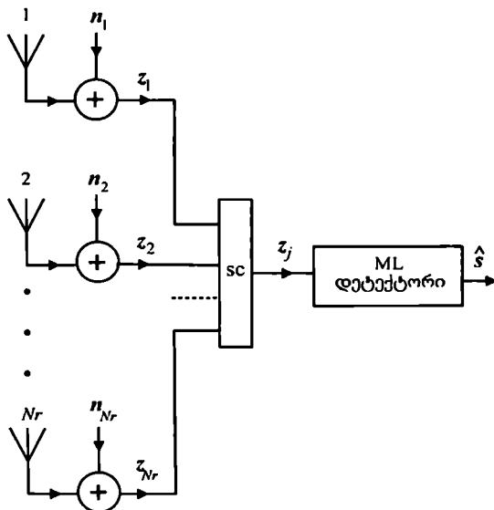
ნახ. 3.4. ამორჩევითი კომბინირების სქემა
