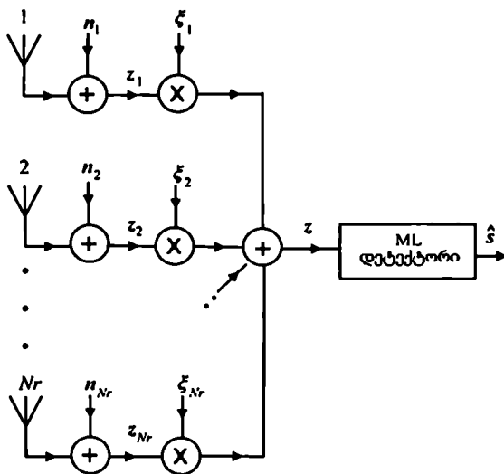
ნახ. 3.7. მაქსიმალური თანაფარდობის კომბინირების სქემა
