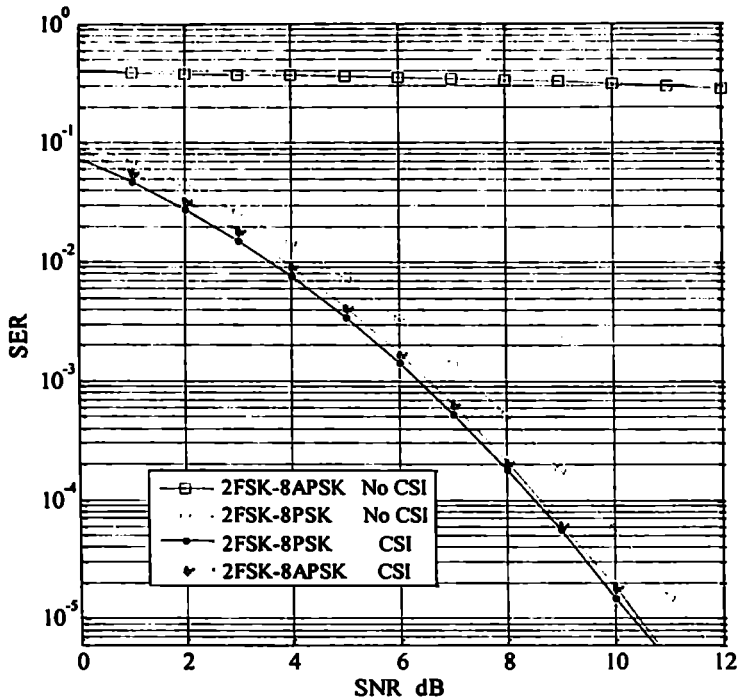
ნახ. 3.13. სიგნალთა SER მაჩვენებლები CSI-ის გამოყენებისას და მის გარეშე MRC კომბინირების სქემისათვის
