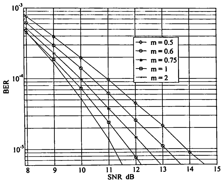
ნახ 4.10. MIMO-SM სისტემის BER მახასიათებლები, როცა a=1 , M=8 , N_t=4 , N_r=8 , S_E=5 ნაკადების არხისათვის
