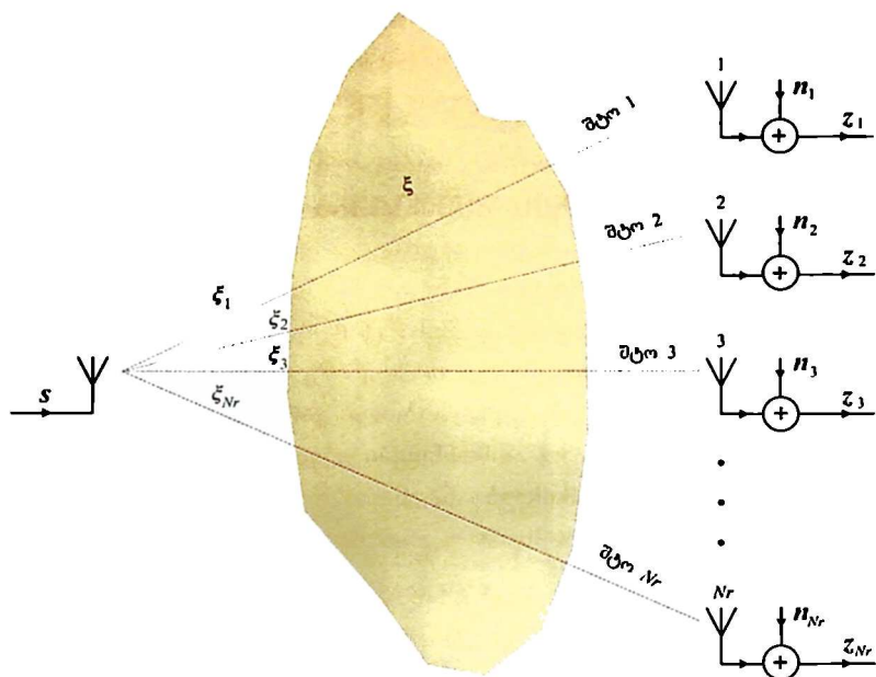
ნახ. 32. სიგნალის მიმორიგებული (პარალელური) მიღების პრინციპული სქემა
