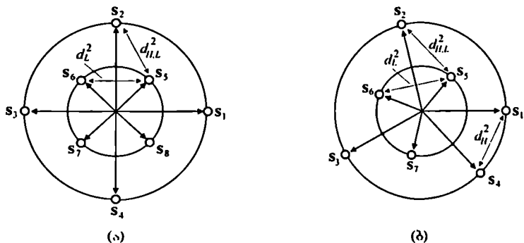
ნახ. 2.5. რეალიზითი (ა) და შეიღობითი (ბ) APSK კონსტელაციები
