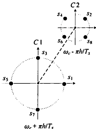
ნახ. 2.10. 4D 2FSK-8APSK კონსტელაციის ინტერპრეტაცია
