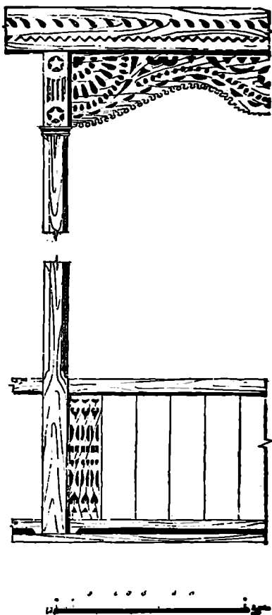
გიორგი ხუტუაშვილის სახლის აივნის დეტალები (ს. ფშაველი)
