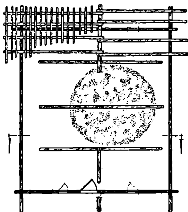
საცხოვრებელი სახლი. სახლი, კრილი და აყარის გეგმა. ს. კახ-ინგილო (ი. ადამიას მიხედვით)
