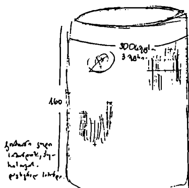
საველე ჩანახატი
