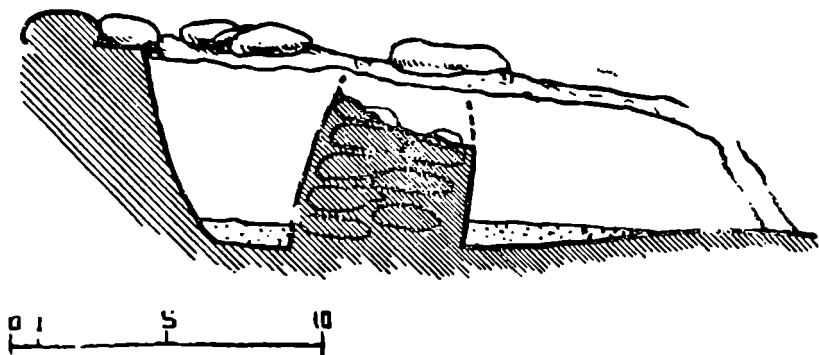
20. უსახელო ბორცვი. კერამიკული ქურის კრლი (არქ. ბ. მკედლიშვილი).
