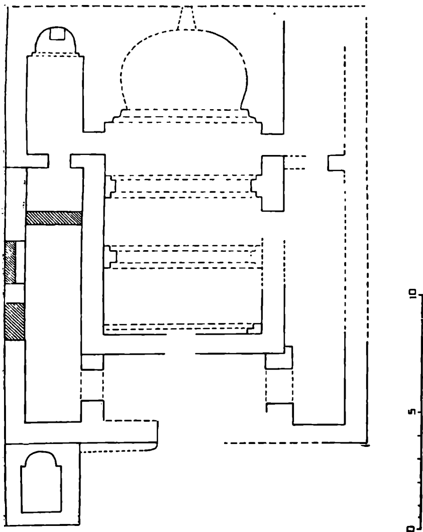
26. საყდრის ყურის ეკლესიის გეგმა (არქ. ბ. შვედლიშვილი).
