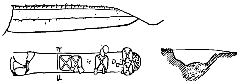
35. კერამიკული ქურის გეგმა და კრილი (არქ. ბ. მკედლიშვილი).
