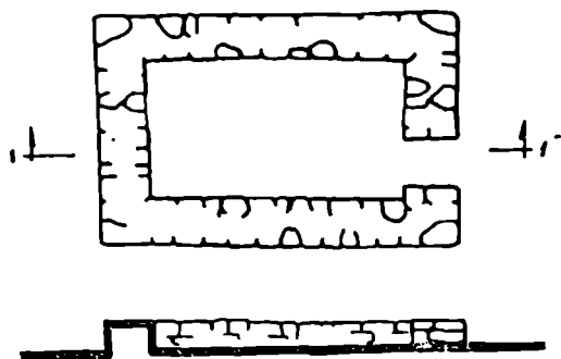
43. ტყის უბნის ნასახლარი № 4, გეგმა და კრილი (აქ.ქ. ნ. ბახტაძე).
