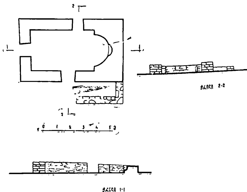
45. ტყის უბნის ეკლესია № 5, გეგმა და ჭრილი (არქ. ნ. ბახტაძე).
