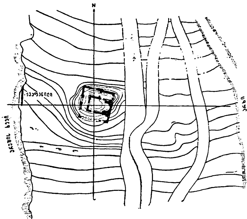
16. უსახელო ბორცი. თვალზომითი გეგმა (არქ. ნ. ბახტაძე).
