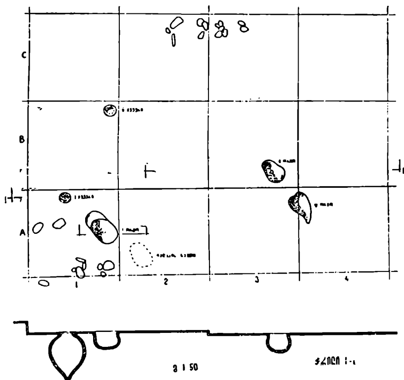
14. „ჩეიდმეტპეტრიანი“. გეგმა (არქ. ნ. ბახტაძე).
