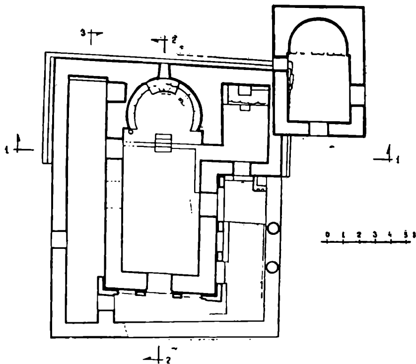
24. მღინარისპირის ეკლესიის გეგმა (არქ. ნ. ბახტაძე).
