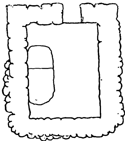
34. საყდრის ყურის ეკლესია. „აკლდამა“. გეგმა დ კრილი (არქ. ბ. მკედლიშვილი).
