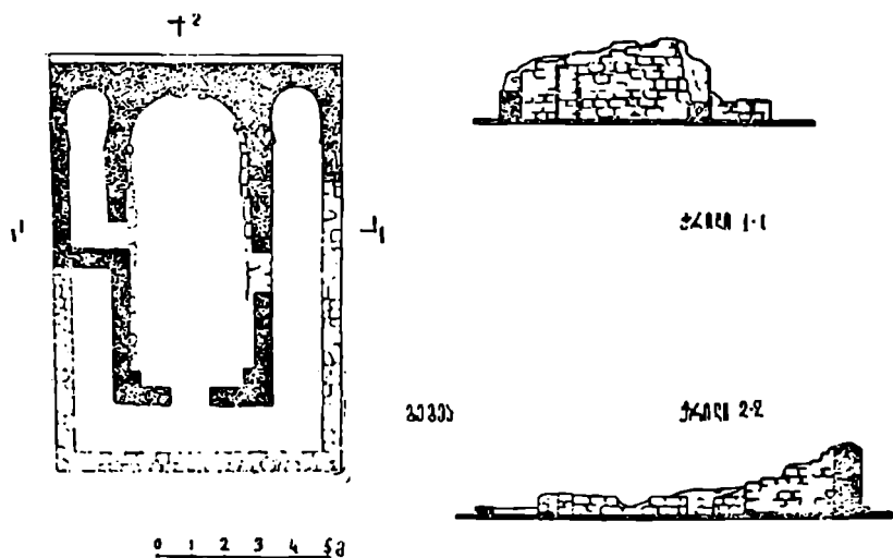
37. ტყის უბანი. ეკლესია № 1, გეგმა და კრილი (არქ. ნ. ბახტაძე).
