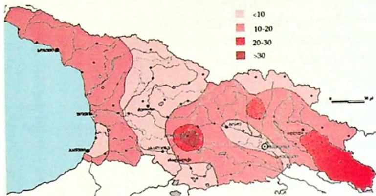
საშუალო ტემპერატურა (°C), % (1999-2010 წწ-ის შედარება 1960 წლამდე მონაცემებთან) მასშტაბი: 1:2 000 000
