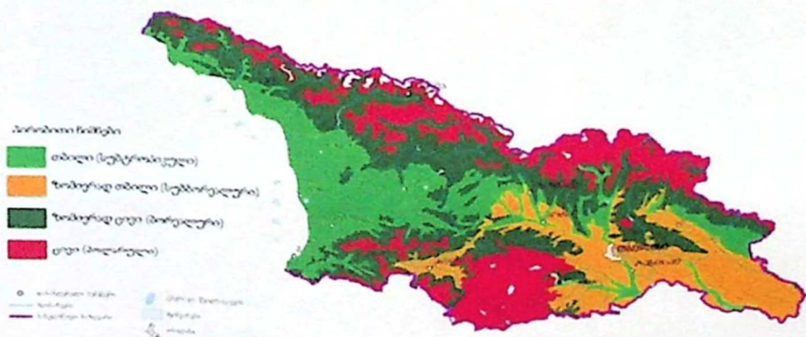
საქართველოს კლიმატის მთავარი თერმული ჯგუფები (ატმოსფერული ტემპერატურათა ჯამი - \Sigma - 10 °C) მასშტაბი 1:1 200 000
