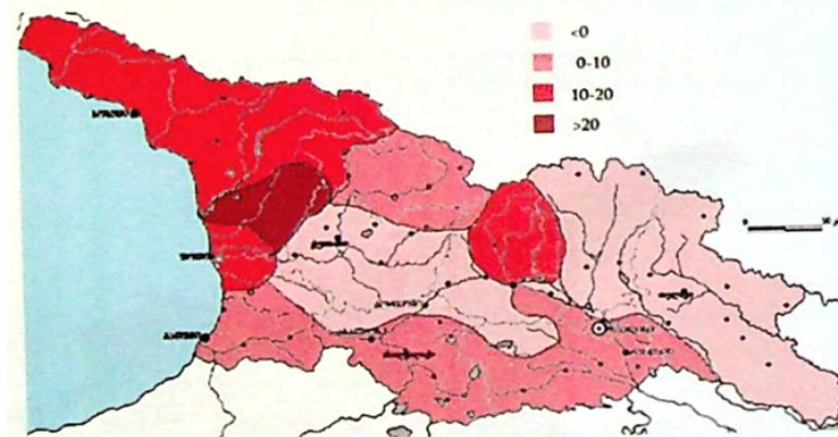
წლიური ნალექები (მმ), % (1999-2010 წწ-ის შედარება 1960 წლამდე მონაცემებთან) მასშტაბი: 1:2 000 000
