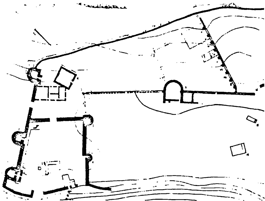
ახალქალაქი. ციტადელის გეგმა.
