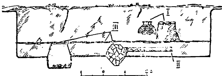
სურ. 17. 36-ე უბნის აღმოსავლეთის თხრილის სიგრძივი კრილი; I. VI—VIII საუკუნეების ნამოსახლარის ნაშთები (კედლის წყობა და ქვევრი. ნაქალაქარის ზედა ფენა); II. ან წ. IV ს. სამარხი; III. ელენისტური ხანის ნამოსახლარის ნაშთები (ნატირანი იატაკი, ქვევრი და მარცვლეულის შესანახი ორმო, რომელშიც ღვება და შეპირილა ჭურჭელია დადასტურებული).
