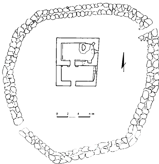
სურ. 65. თრიალეთი. თეჯისი /ლიპი. სამლოცველოს გეგმა (შ. მელიქიძის ანაზომი).
