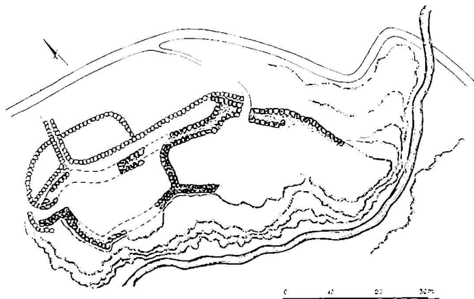
სურ. 140. თრიალეთი. აშკალა. პირველი „ციკლოპური“ სიმაგრე. გეგმა (შეადგინეს შ. მელიქიძემ და გ. ნარიშკინი).
