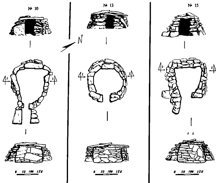
სურ. 83. ჯავახეთი. შაორი. გზის გასწვრივ არსებული მცირე ზომის სენაკები (შ. მელიქიძის ჩანახატი).
