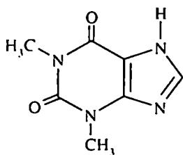
თეოფილინი
