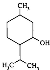
მენტოლი
