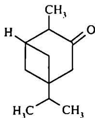
ბ-ტუიონი
