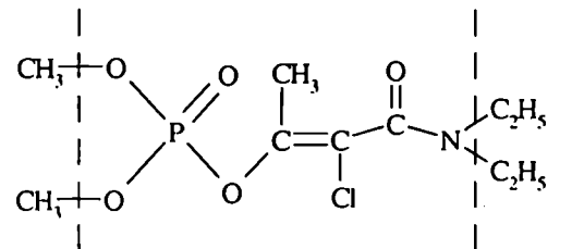
N-ალკილური ჯგუფები
