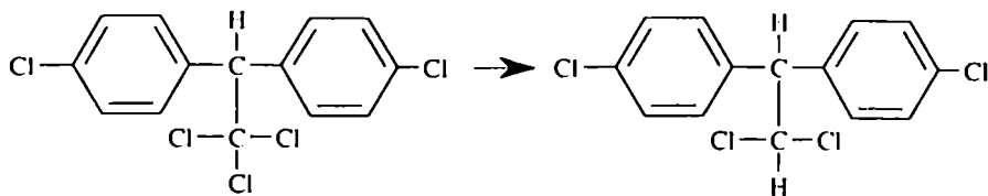
დღტ
