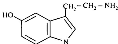
სეროტონინი
