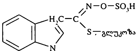
გლუკობრასიცინი
