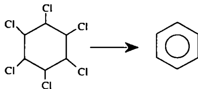
ბენზოლი
