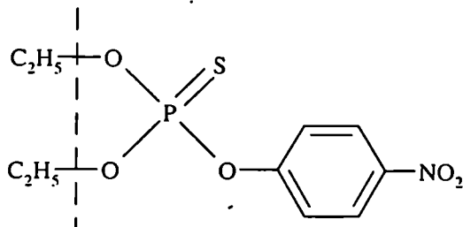
პარათიონი
