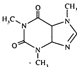
კოფეინი
