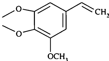
მირისტინი
