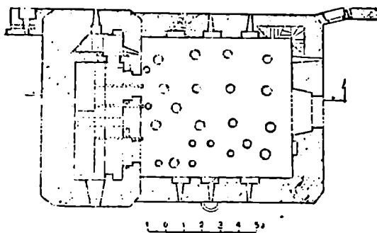
სურ. 59. ზემო ხოდაშენი. კოშკი მარნით. პირველი სართულის გეგმა
