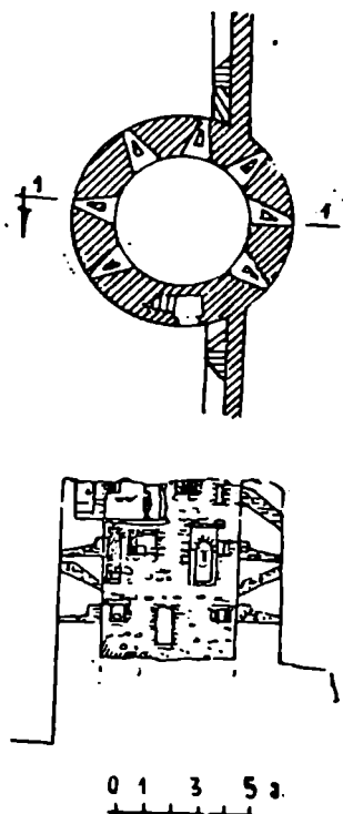
სურ. 15. სილნალი. ციხის აღმოსავლეთის კოშკის გეგმა და განაკვეთი
