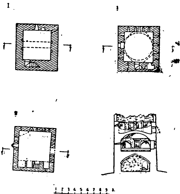
სურ. 43. ნორიო „ცოფურაანთ კოშკი“. განაკვეთი და გეგმები
