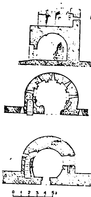
სურ. 30. ყვარელი. ციხის დასაუღეთის კოშკის განაკვეთი და გეგმები
