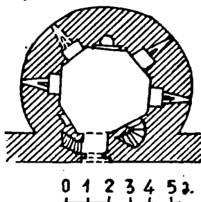
სურ. 42. ბანში. სამხრეთის კოშკის გეგმა
