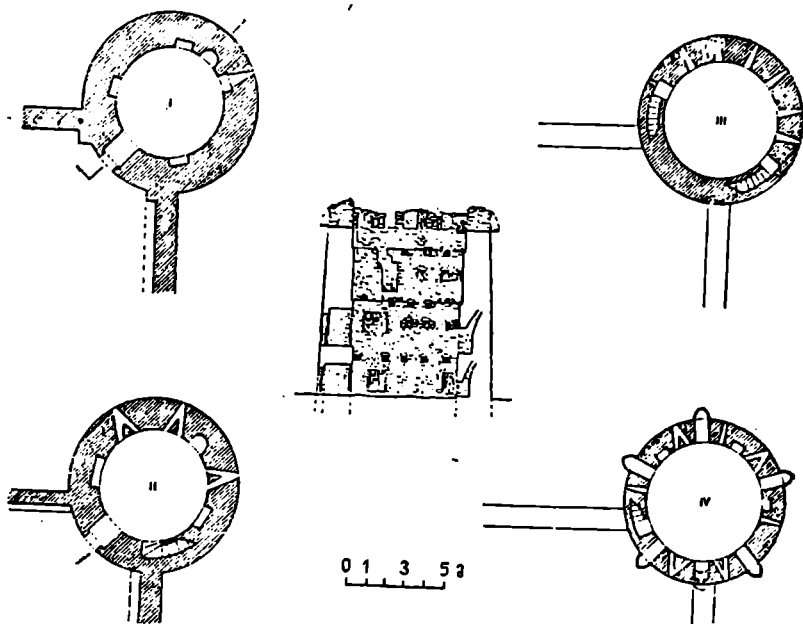
სურ. 36. ნაფარეული. ციხის ჩრდილო-დასავლეთის კოშკის გეგმები და განაკვეთი
