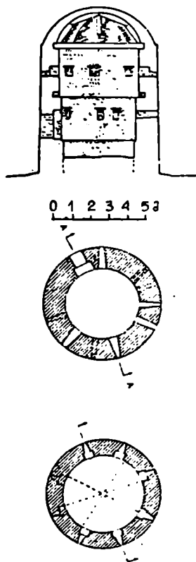
სურ. 57. სოფ. გიორგი წმინდა. კოშკის განაკვეთი და გეგმები
