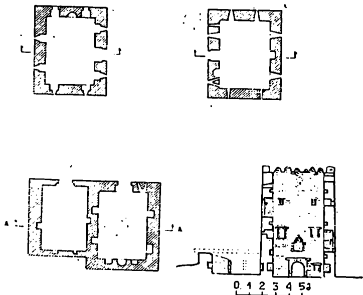
სურ. 44. ნორიო. „ქვეერაანთ კოშკი“. გეგმები და განაკვეთი
