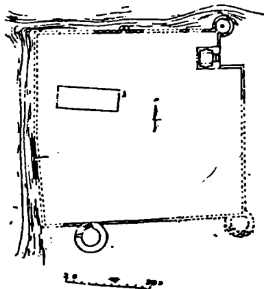
სურ. 40. ხაშში. ციხის გეგმა
