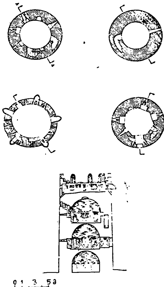
სურ. 55. პატარძელის ბილანიშვილების კოშკი. განაკვეთი და გეგმები
