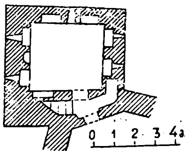
სურ. 22. რუისპირი. ჩრდილო-აღმოსავლეთის კოშკის გეგმა
