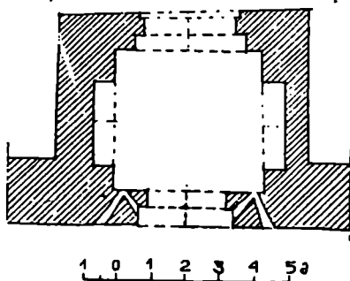
სურ. 37. შილდა. ციხის შესასვლელი კოშკის გეგმა
