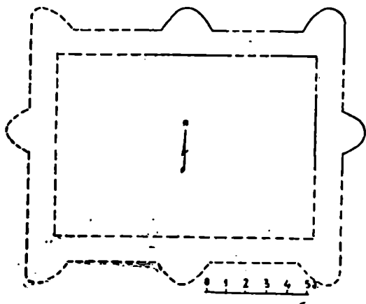
სურ. 9. ჩაილური. კოშკის პირველი სართულის სქემატური გეგმა
