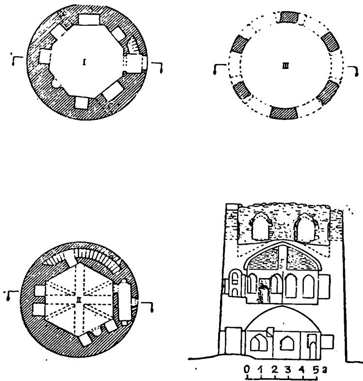
სურ. 50. კისისხევი. კოშკის გეგმები და განაკვეთი
