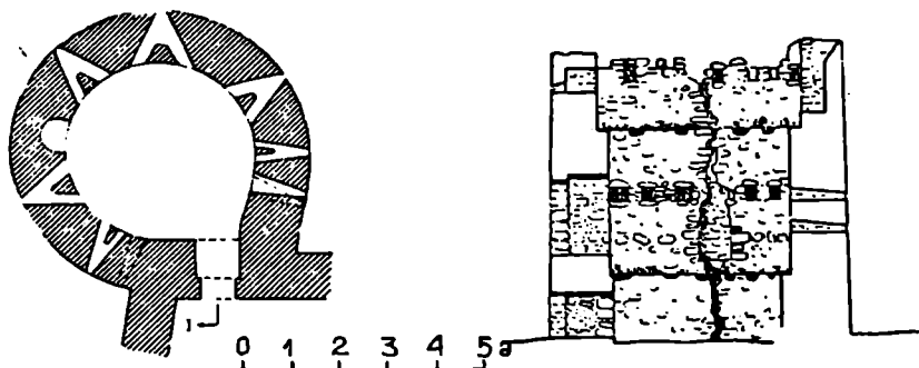
სურ. 8. ჩაილური. ჩრდილო-დასავლეთის კოშკის გეგმა და განაკვეთი
