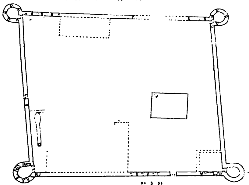
სურ. 16. მატანის ციხის გეგმა
