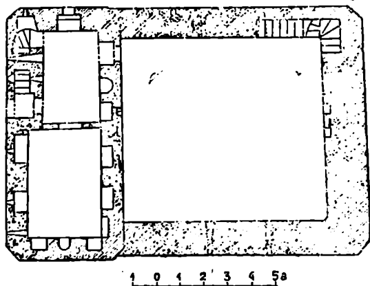
სურ. 60. ზემო ხოდაშენი. კოშკი მარნით. მეორე სართულის გეგმა
