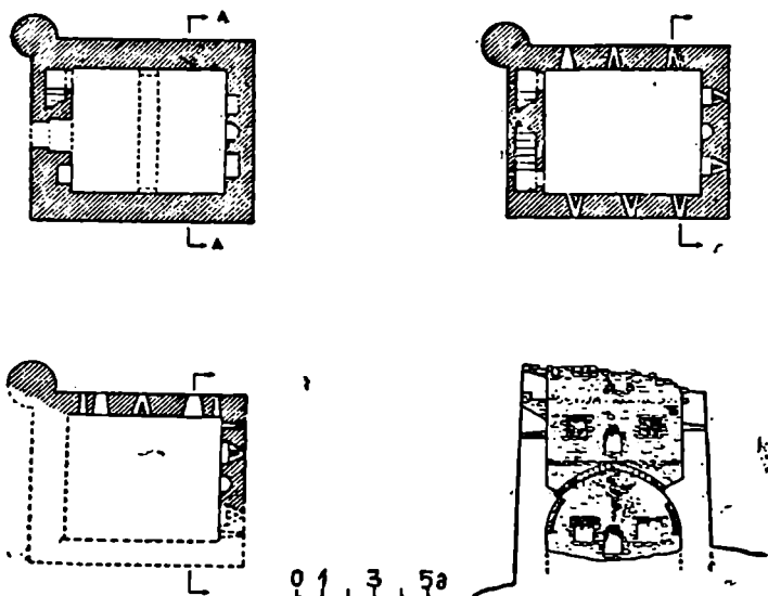
სურ. 46 ლალისყური. „ტალის-ციხის“ განაკვეთი და გეგმები
