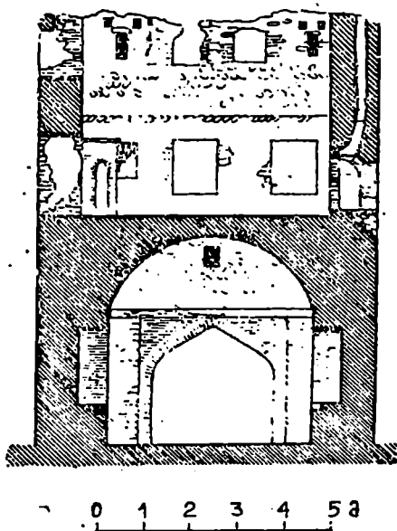
სურ. 38. შილდა. ციხის შესასვლელი კოშკის განაკვეთი
