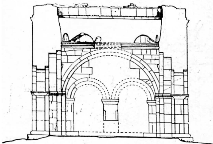
სურ. 70. სამრეკლოს განაკვეთი. ანაზომი არქ. რ. გვერდწითელისა
