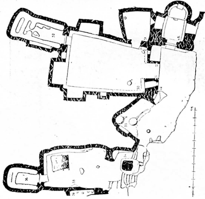
სურ. 59. „სადარბაზოს“ ჯგუფის გეგმა ანბოში არქ. კ. მელითაურისკ
