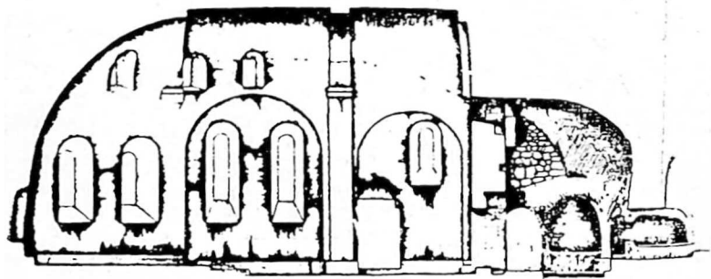
სურ. 36. განაკვეთი სიღრმეზე. ანაზომი არქ. კ. მელითაურისა.
