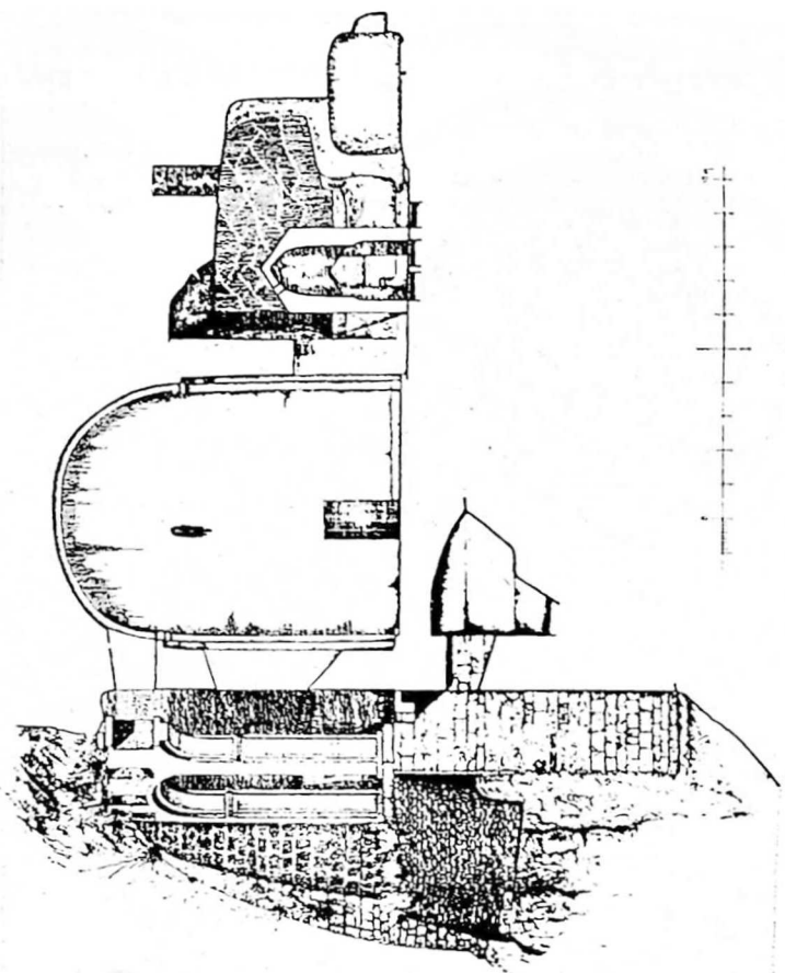
სურ. 35. განაკვეთი სიღრმეზე. ანაზომი არქ. კ. მელითაურისა
