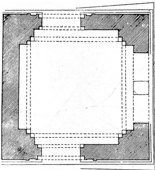
სურ. 69. სამრეკლოს გეგმა. ანაზომი არქ. რ. გვერდწითელისა
