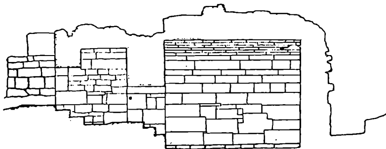
სურ. 2. აკლამა. სიგრძივი ჭრილი.
