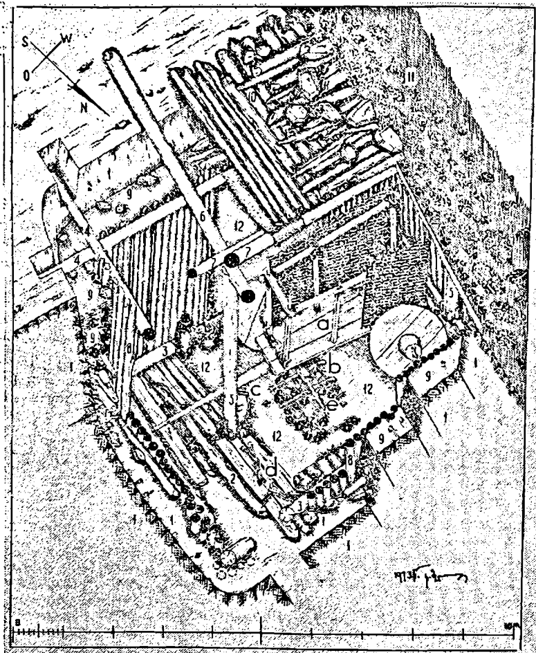
სურ. 9. გორასმარხი 5. ხის აკლდამის რეკონსტრუქცია (ჟ. მელითაურის მიხედვით)
