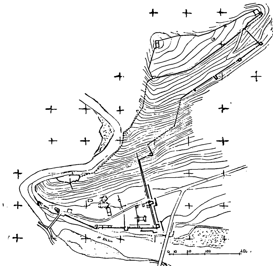
ციხეგოჯი-ნოქალაქევი. ნაქალაქარის გეგმა
