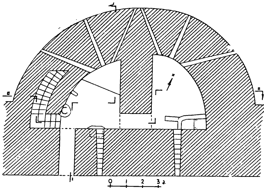
ურბნისი. ალიზის კოშკის გეგმა
