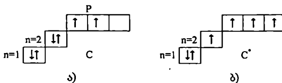
ნახ.4. ა) ნახშირბადი ნორმალურ მდგომარეობაში
