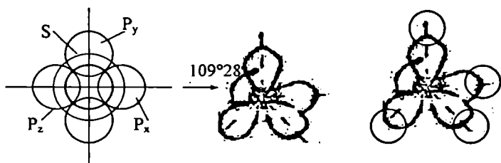
ნახ.5. ნახშირბადატომის ორბიტალების SP^3 ჰიბრიდიზაცია
