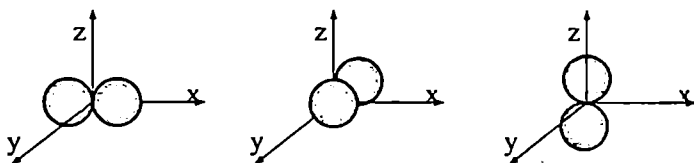
ნახ.3. P_x , P_y , P_z ატომური ორბიტალები
