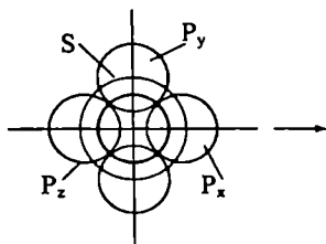
ნახ.7. ნახშირბადატომის ორბიტალების SP^3 ჰიბრიდიზაცია
