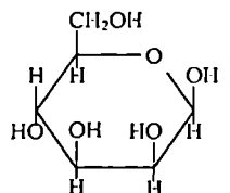
β, D(+) მანოპირანოზა
