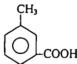
მ-ტოლუილმჟავა (მ-მეთილბენზოის მჟავა)
