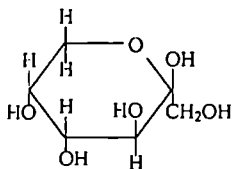
β D(-) ფრუქტოპირანოზა
