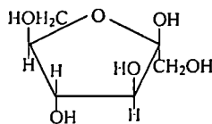
β D(-) ფრუქტოფურანოზა
