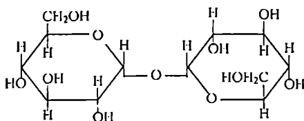
ტრეგალოზა ( \alpha D-გლუკოპირანოზიდი) - \beta D - გლუკოპირანოზიდი
