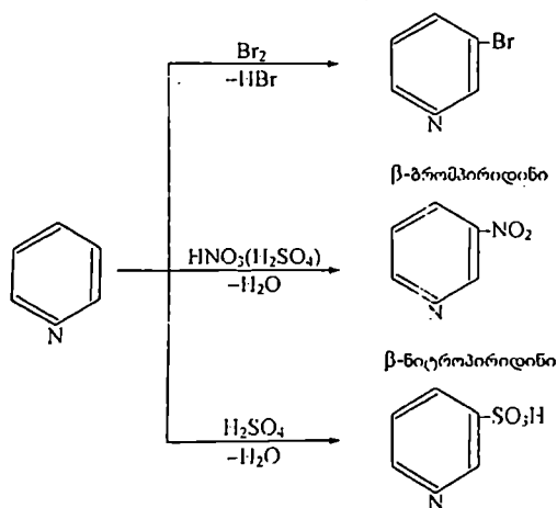
პირიდინ- \beta -სულონომაჟა
