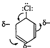
ქლორბენზოლის ელექტრონული სრუქტურა
