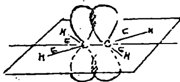
ნახ.9. π-ბმის წარმოქმნა ეთილენის მოლეკულაში
