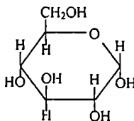
\alpha D გლუკოპირანოზა
