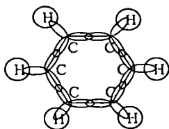
C-ატომების ჰიბრიდული σ-ორბიტალები ბენზოლის მოლეკულაში
