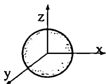
ნახ.2. S-ატომური ორბიტალი
