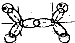
ნახ.8. σ-ბმები ეთილენის მოლეკულაში
