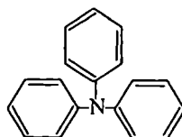
ტრიფენილამინი (მესამეული ამინი)
