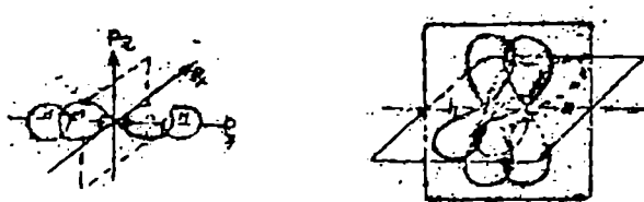
ნახ.11. \sigma და \pi ბმის წარმოქმნის სქემა აცეტილენის მოლეკულაში
