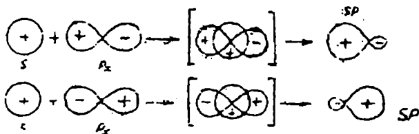
ნახ.10. ნახშირბადატომის ორბიტალების ჰიბრიდიზაცია
