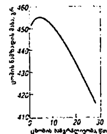
ნახ.16. ცომის ნამზადის მასის ცვლილება ცხობის პირველ სტადიაზე დატენიანებული საკანში ცხობის დროს
