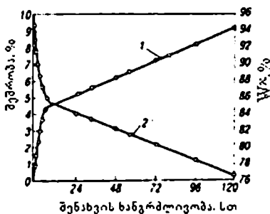
ნახ. 25. პურის შემორობის (1) და შრობის (2) მრუდები
