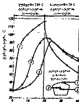
ნახ.23. ცომის ნაშადის ტემპერატურული ველი ცხოვის მომენტში და ღუმელიდან გამოღების შემდეგ
