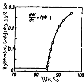
ნახ. 26. პურის შრობის სიჩქარის მრუდი
