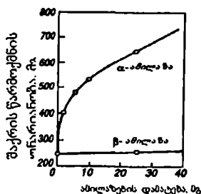
ნახ. 2 \alpha - და \beta -ამილაზასაგაღვლენა ხორბლის ფქვილის შაქრის წარმოქმნის უნარზე
