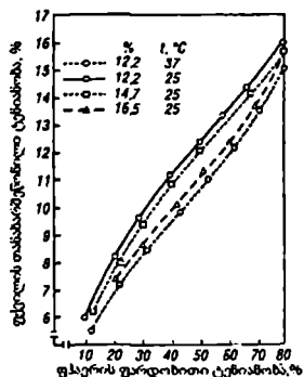
ნახ. 4 ფქვილის თანასწორობითი ტენიანობის დამოკიდებულება ჰაერის ტენიანობასა და ტემპერატურაზე
