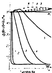
ნახ.18. ცომის ნამზადის ცალკეულ ფენებში ტენიანობის ცვლილება (მრუდების შემოყრისა იგივეა რაც ნახ.10-ში)
