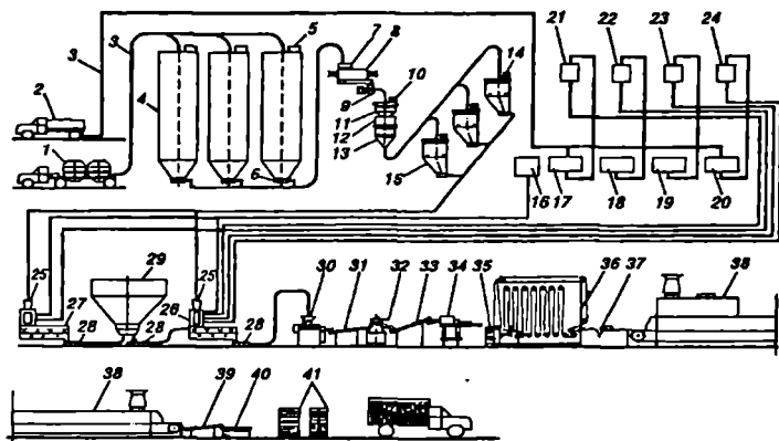
ნახ.1 პურის წარმოების სქემა
